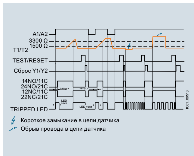
3RN2012-.B.30, 3RN2013: Сброс через кнопку ТЕСТ/СБРОС или внешнюю кнопку
