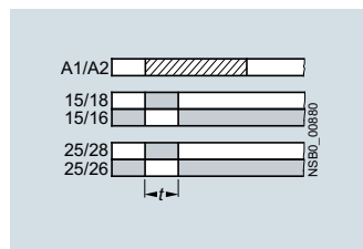
E 3RP2005-B с проскальзывающим нормально открытым контактом
