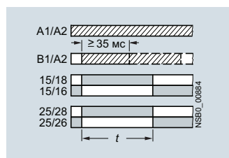
F 1) 7PV1508-1B с формированием импульсов по управляющему сигналу (создание импульса на выходе независимо от продолжительности возбуждения)
