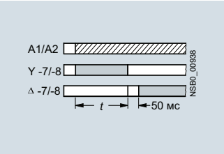
3RT1926-2G Функция «звезда-треугольник» 1 нормально открытый контакт с задержкой, 1 нормально открытый контакт
