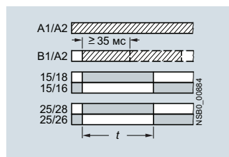
G¹) 3RP2005-B с формированием импульсов по управляющему сигналу (создание импульса на выходе независимо от продолжительности возбуждения)
