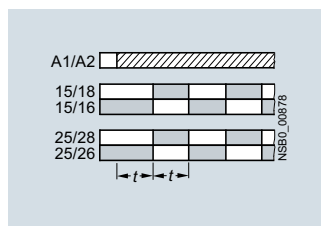
D 3RP2005-B с мигающим режимом, начало с паузы (импульс/пауза 1:1)
