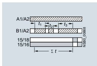
G 1) 7PV1508-1A аддитивная задержка на включение по управляющему сигналу
