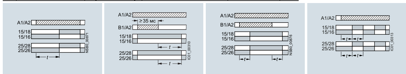
A с задержкой на включение
