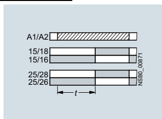
3RP2525..W30, 2 П, с задержкой на включение
