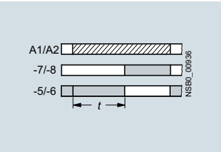
3RT1926-2E с задержкой на включение
