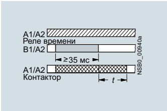
3RT1926-2D с задержкой на выключение по управляющему сигналу (варистор не встроен)
