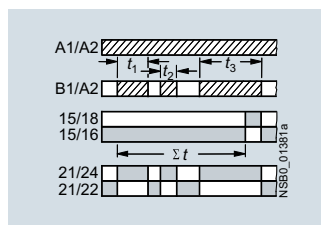
H•¹) 3RP2005-B аддитивная задержка на включение по управляющему сигналу и с мгновенным срабатыванием
