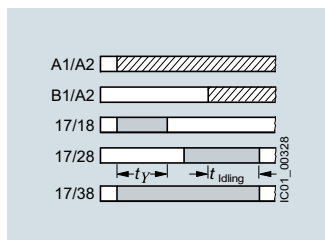
3RP2560..SW30, 3 НО, функция «звезда-треугольник» с функцией выбора (Idling)
