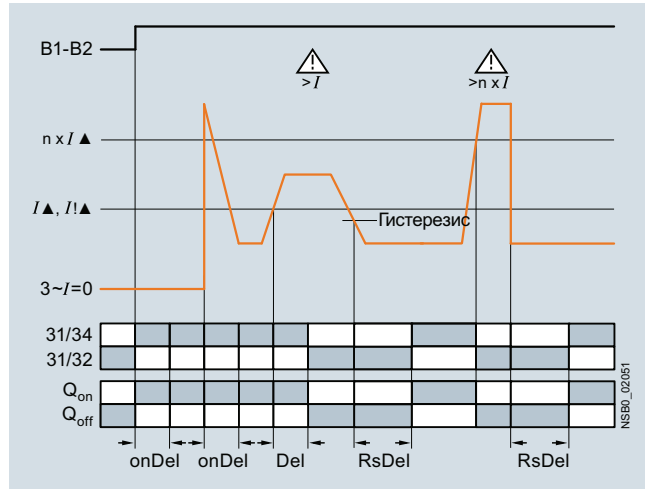
Превышение тока
