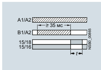
F 1) 3RP2005-A с проскальзывающим размыкающим контактом по управляющему сигналу
