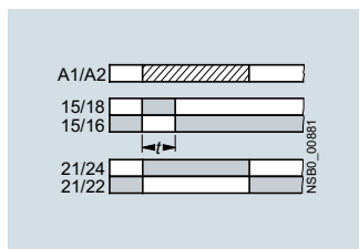
E• 3RP2005-B с проскальзывающим нормально открытым контактом и с мгновенным срабатыванием
