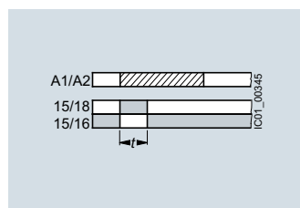
E с проскальзывающим нормально открытым контактом, интервальное реле
