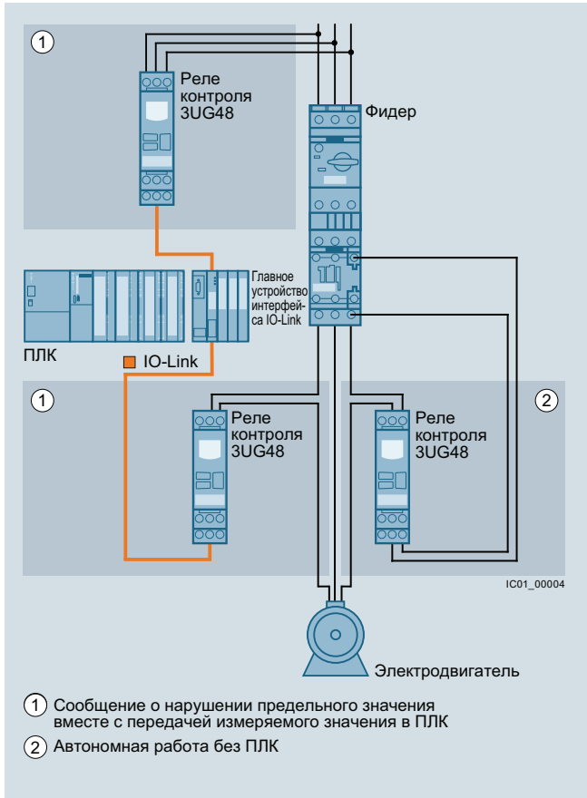
Реле контроля для IO-Link
