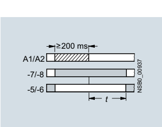
3RT1926-2F с задержкой на выключение не по управляющему сигналу
