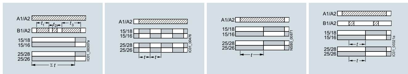
I аддитивная задержка на включение по управляющему сигналу
