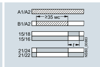
F•¹) 3RP2005-B с проскальзывающим размыкающим контактом и с мгновенным срабатыванием
