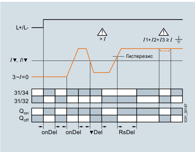
Понижение тока с контролем тока утечки
