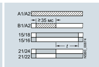
B•¹) 3RP2005-B с задержкой на выключение по управляющему сигналу и с мгновенным срабатыванием
