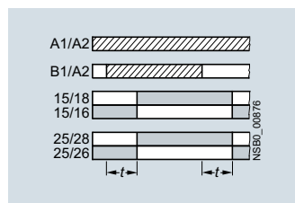
C¹) 3RP2005-B с задержкой на включение и на выключение по управляющему сигналу ( t = t_{an} = t_{ab} )
