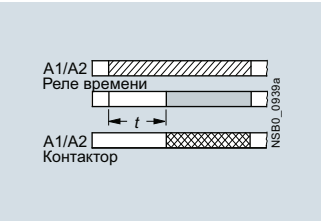
3RT1926-2C с задержкой на включение двухжильное исполнение (варистор встроен)
