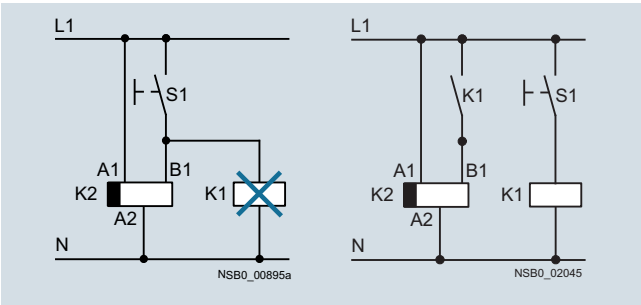
Схемы соединений
