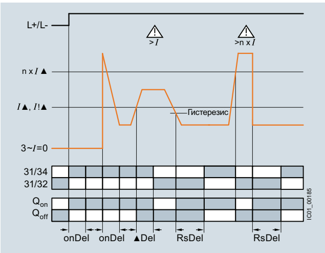
Превышение тока
