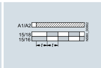
C 7PV1508-1A с мигающим режимом, пуск с паузы (импульс/пауза 1:1)
