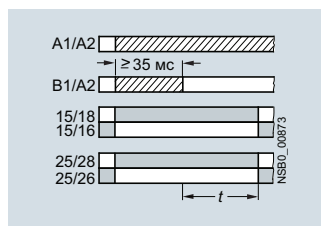
B¹) 3RP2005-B с задержкой на выключение по управляющему сигналу
