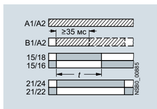
G•¹) 3RP2005-B с формированием импульсов по управляющему сигналу и с мгновенным срабатыванием (создание импульса на выходе независимо от продолжительности возбуждения)
