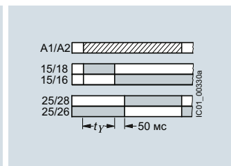
3RP257..NW30, 2 НО, функция «звезда-треугольник»
