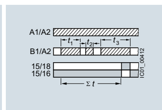
H аддитивная задержка на включение, без задержки, с выключением по управляющему сигналу
