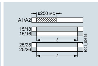
3RP2540..B.30, 2 П, устойчиво к прохо- ждению сигнала, с проскальзываю- щим нормально открытым контактом (O) 1)
