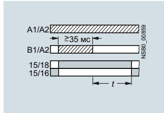
B 1) 3RP2005-A с задержкой на выключение по управляющему сигналу
