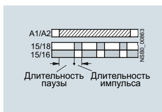
- 7PV1558 пульсация, пуск с паузы (длительность паузы, длительность импульса и временные диапазоны можно настраивать отдельно в каждом случае)
