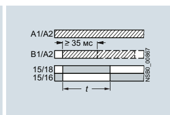
F 1) 7PV1508-1A с формированием импульсов по управляющему сигналу (создание импульса на выходе независимо от продолжительности возбуждения)
