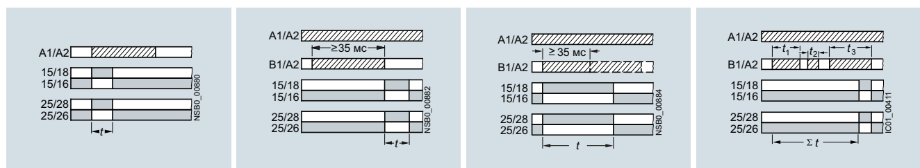
E с проскальзывающим нормально открытым контактом, интервальное реле
