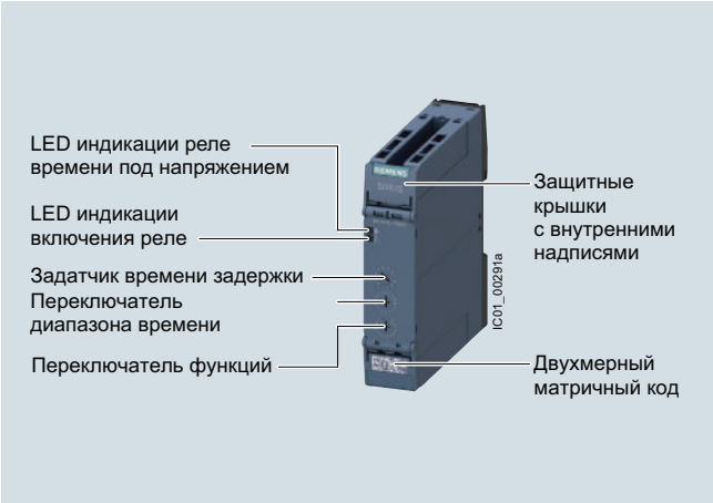
Реле времени SIRIUS 3RP25
