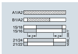
C•¹) 3RP2005-B с задержкой на включение и на выключение по управляющему сигналу и с мгновенным срабатыванием ( t = t_{an} = t_{ab} )
