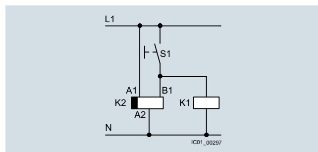
Схема соединений
