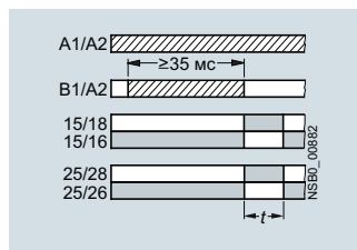
F¹) 3RP2005-B с проскальзывающим размыкающим контактом
