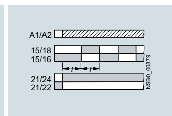
D• 3RP2005-B с мигающим режимом, начало с паузы (импульс/пауза 1:1) и с мгновенным срабатыванием
