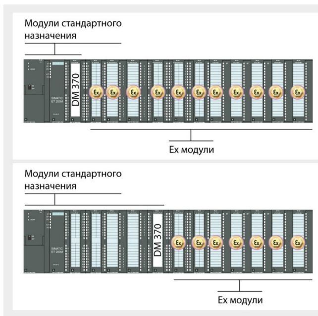
Ex перегородка
