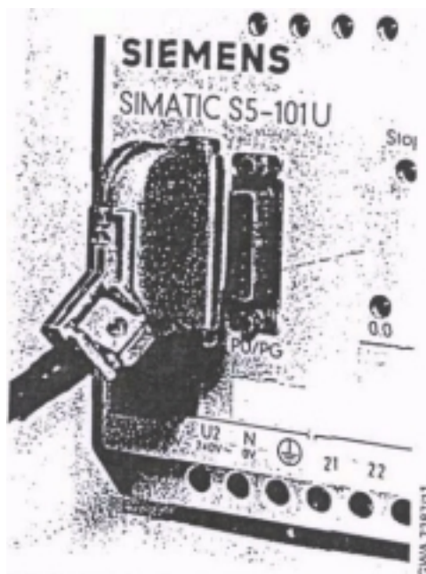
Рис. 2-3. Подключение ОП 393 к S5-101U
