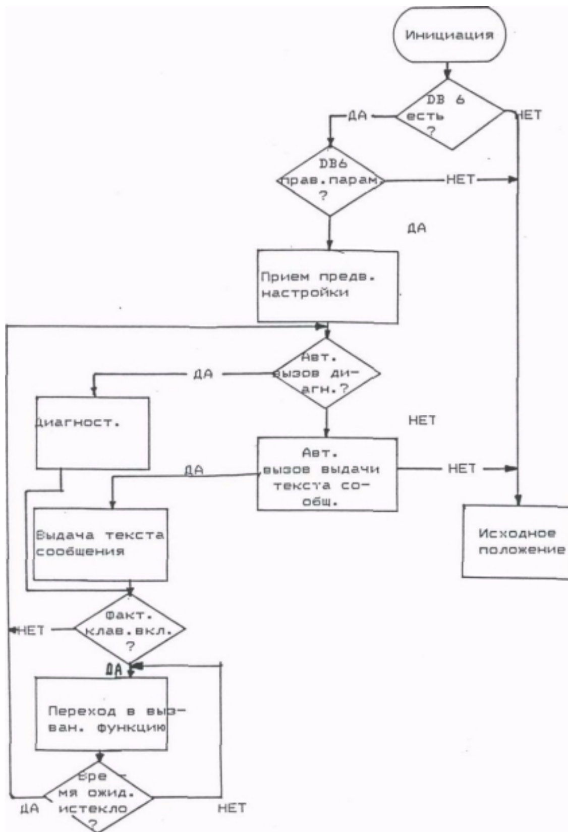
Рис. 2.6 Диаграмма цикла: принцип действия ОР 393
