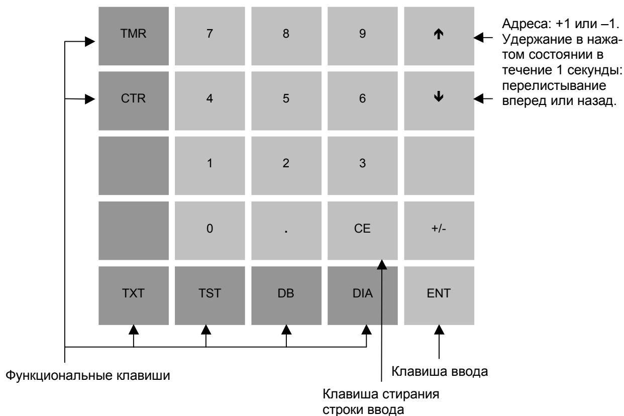
Рис. 2-4. Клавиатура ОП 393-II
