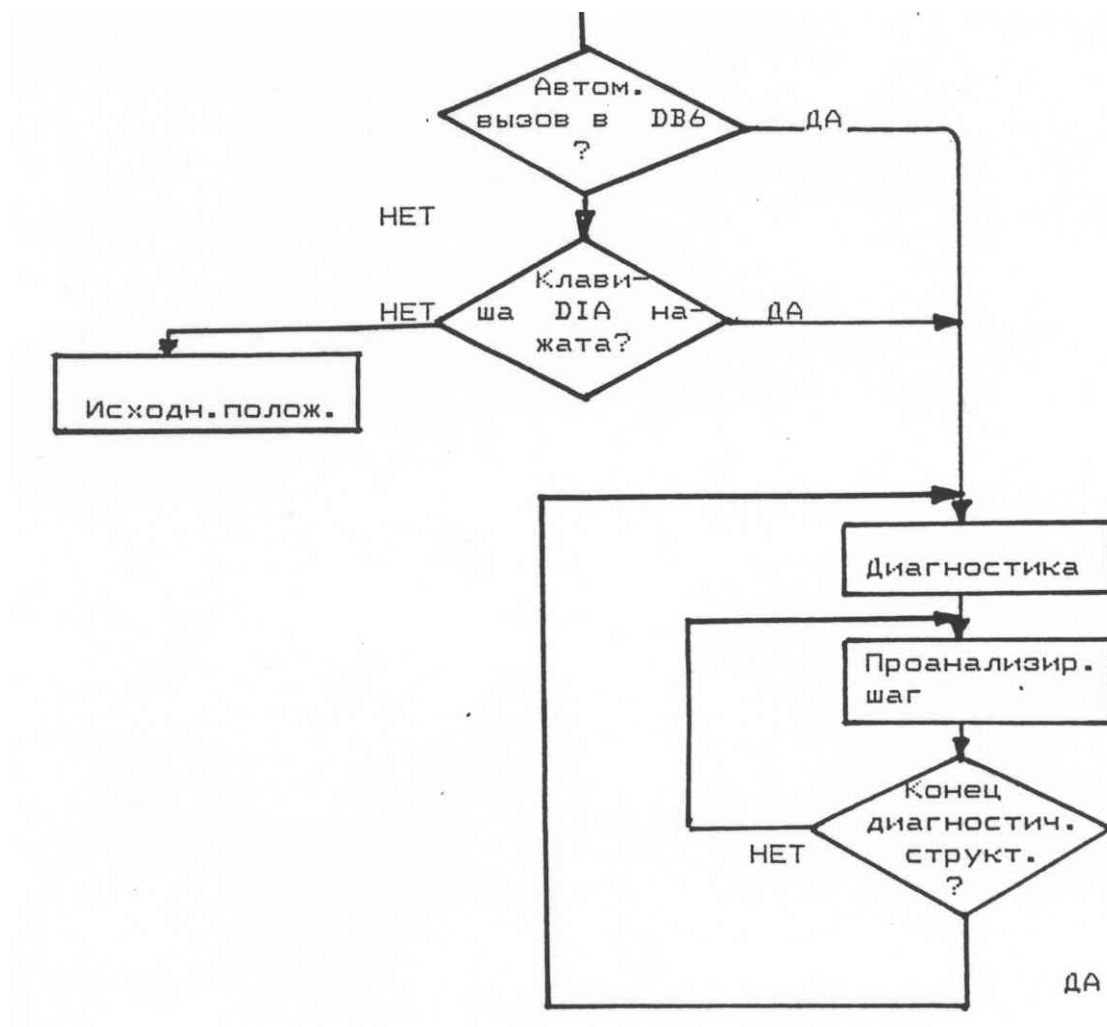
Рис. 7.2 Диаграмма цикла: вызов диагностики
