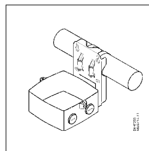
Монтаж на горизонтальной трубе
