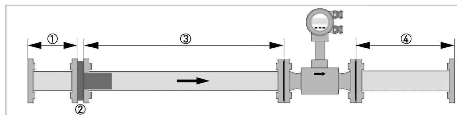
Рис. 3-9: Выпрямитель потока
