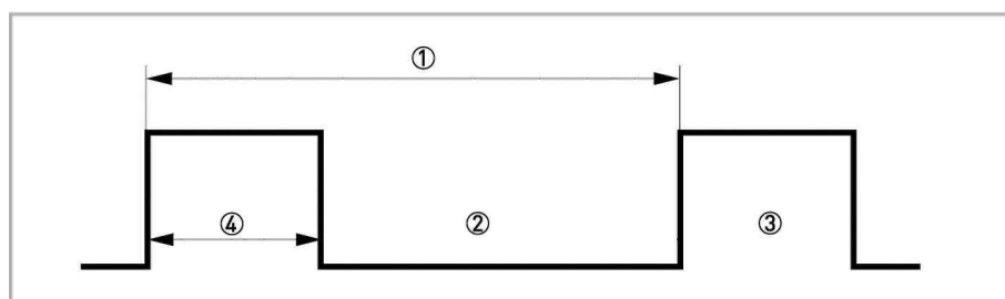
Рисунок 4-3: Импульсный выход:
