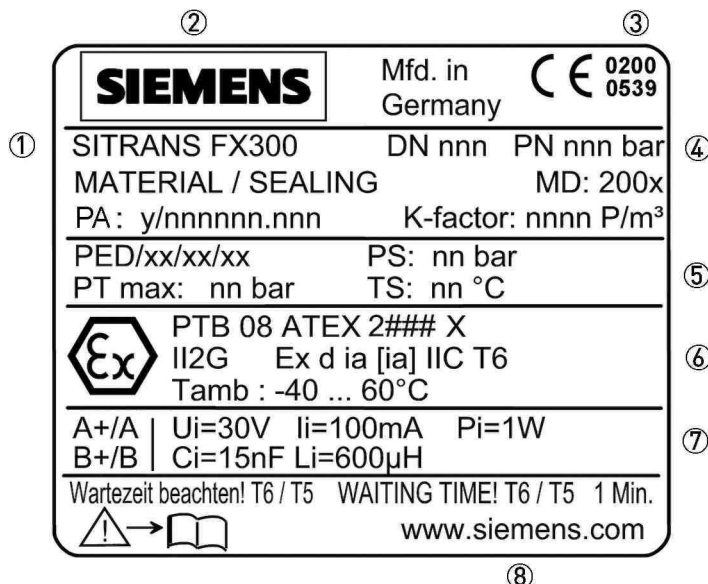
Рис. 2-5: Пример паспортной таблички
