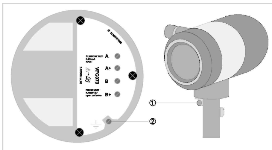
Рисунок 4-5: Заземление
