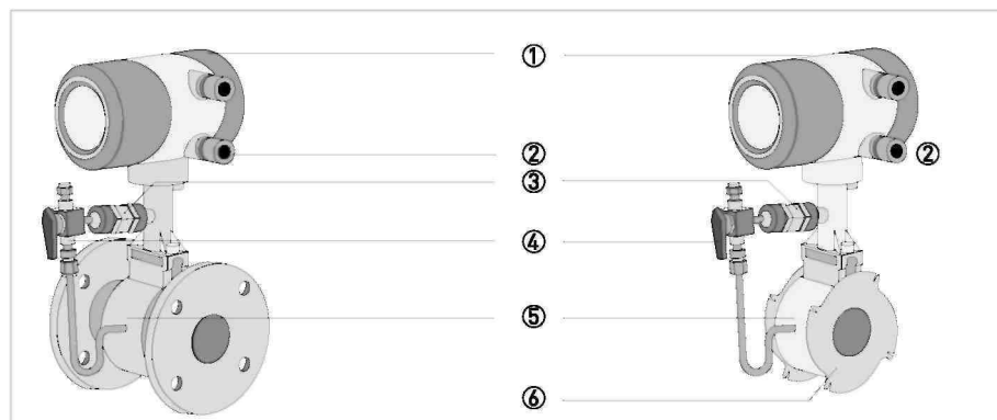
Рис. 2-4: Описание прибора
