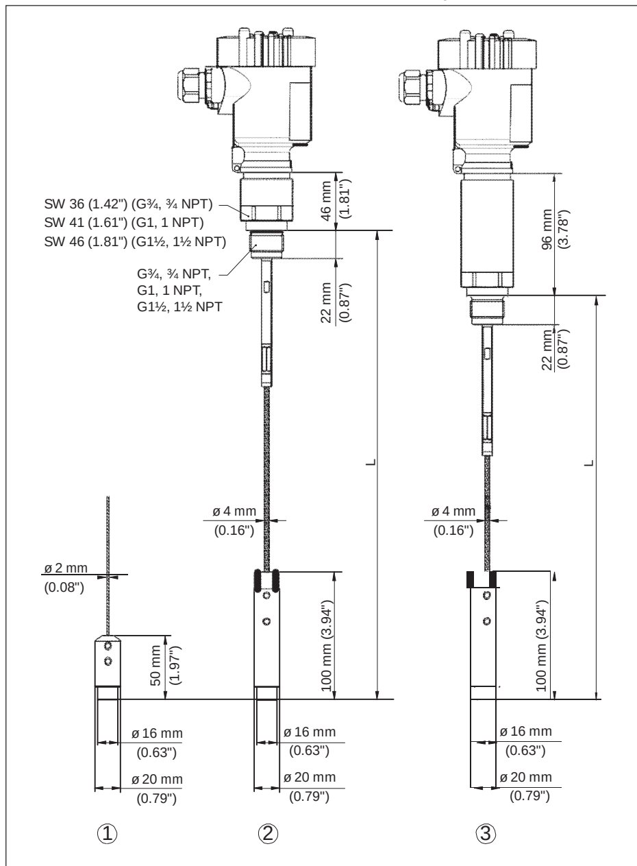
Рис. 60: SITRANS LG250, резьбовое исполнение с натяжным грузом (все натяжные грузы с резьбой M8 для рым-болта)
