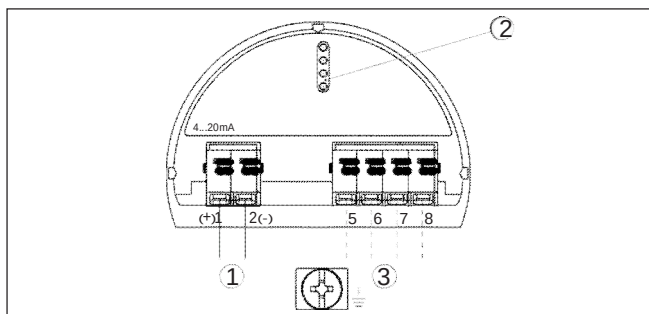
Рис. 20: Отсек электроники (двухкамерный корпус)
