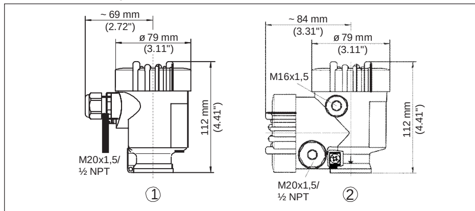
Рис. 55: Корпуса в исполнении IP 66/IP 68 (0,2 bar) - с установленным модулем индикации и настройки корпус выше на 9 мм/0.35 in
