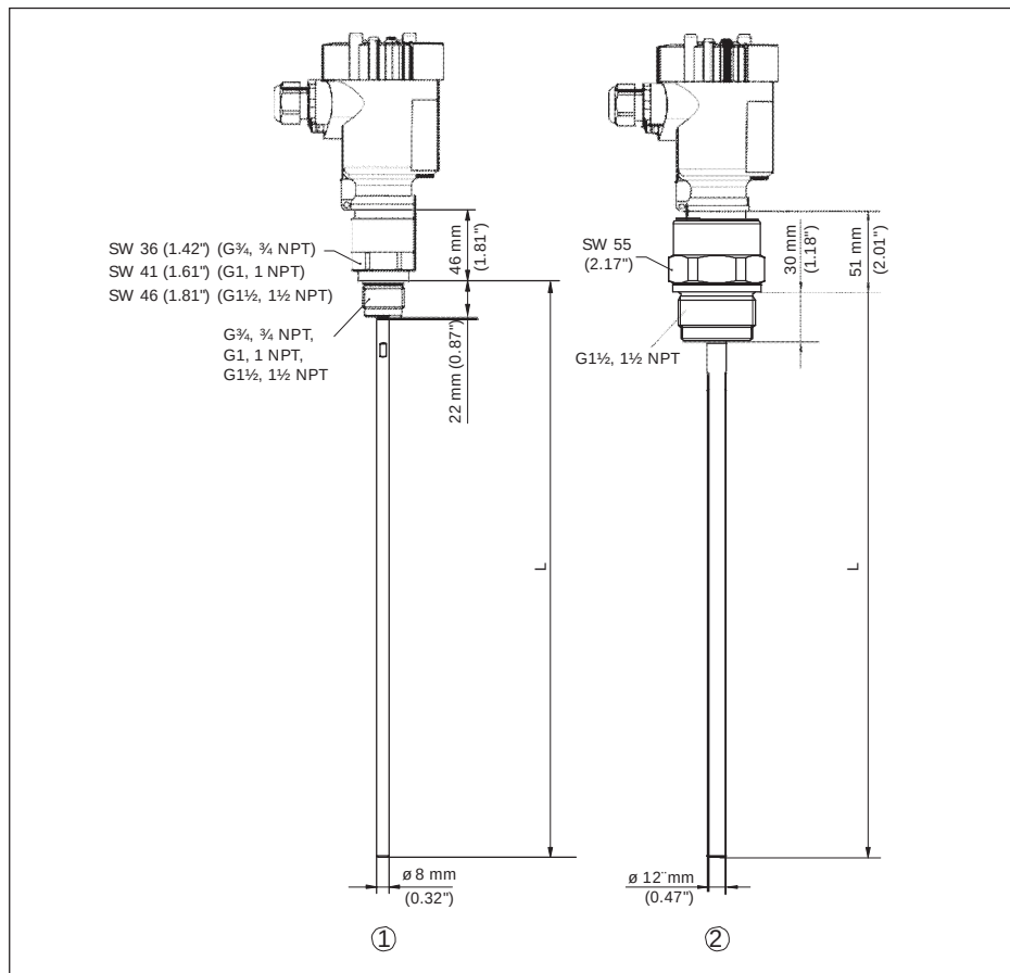
Рис. 62: SITRANS LG250, резьбовое исполнение
