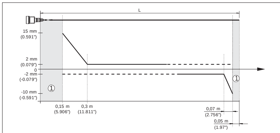
Рис. 49: Погрешность измерения SITRANS LG250 в стержневом исполнении (продукт - масло)
