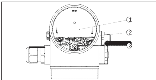
Рис. 22: Отсек электроники - вид сверху
