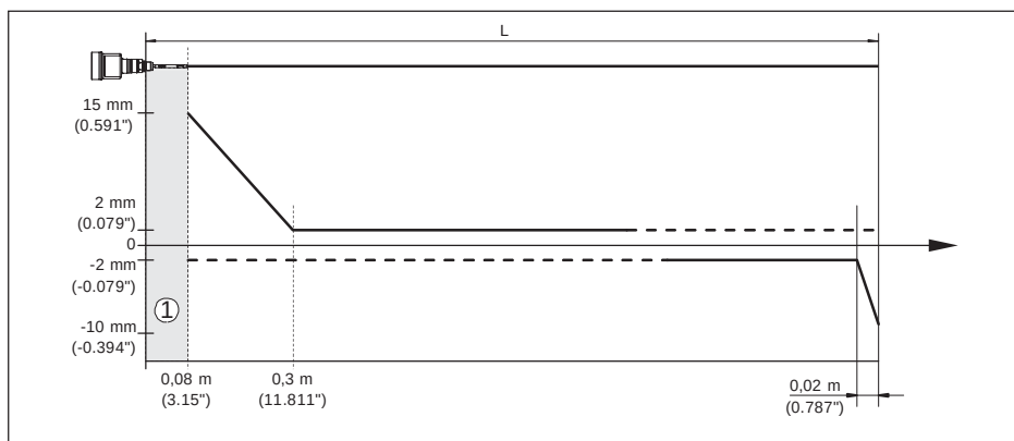
Рис. 48: Погрешность измерения SITRANS LG250 в стержневом исполнении (продукт - вода)
