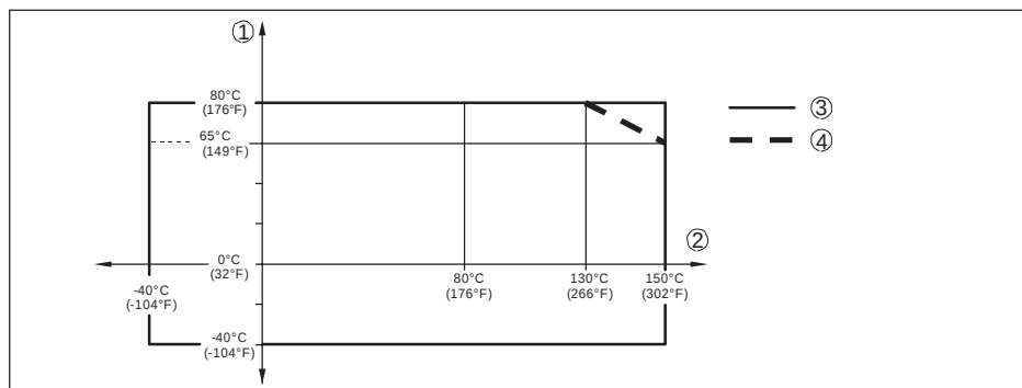
Рис. 53: Температура окружающей среды - температура процесса, стандартное исполнение
