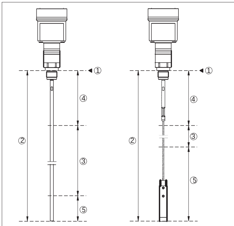
Рис. 47: Диапазоны измерения - SITRANS LG250
