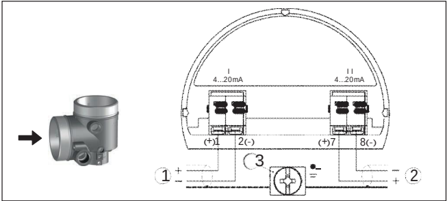
Рис. 25: Отсек подключения в двухкамерном корпусе, дополнительная электроника - второй токовый выход
