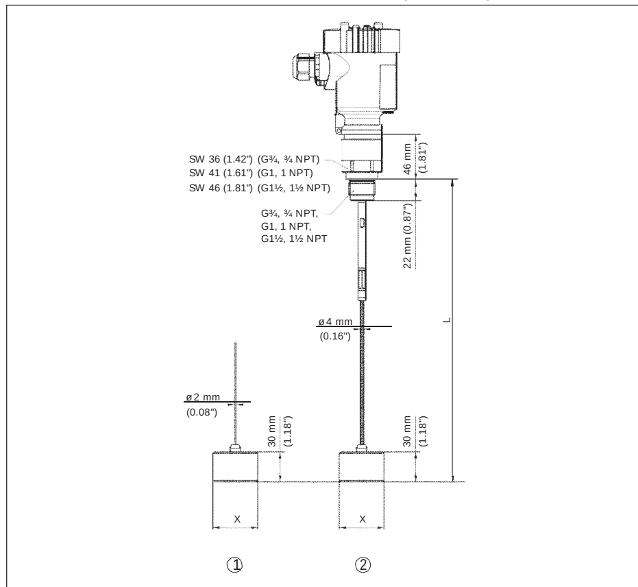
Рис. 61: SITRANS LG250, резьбовое исполнение
