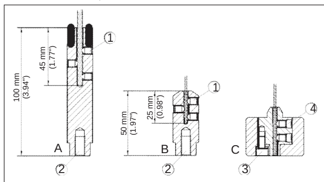
Рис. 46: Укорачивание измерительного троса
