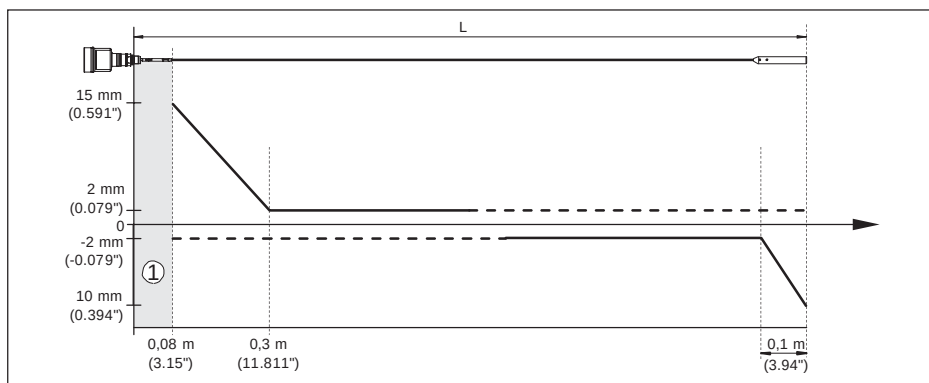
Рис. 50: Погрешность измерения SITRANS LG250 в тросовом исполнении (продукт - вода)
