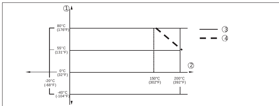
Рис. 54: Температура окружающей среды - температура процесса, исполнение с температурной вставкой
