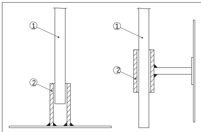
Рис. 13: Фиксация измерительного зонда
