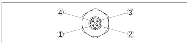
Рис. 23: Разъем - вид сверху
