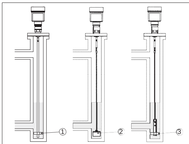
Рис. 12: Положение центрирующей звездочки или центрирующего груза
