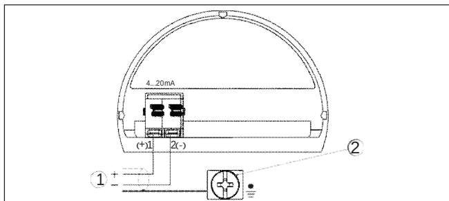
Рис. 21: Отсек подключения (двухкамерный корпус Ex d)
