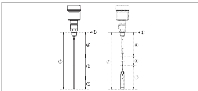
Рис. 3: Диапазоны измерения - SITRANS LG250
