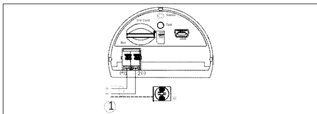
Рис. 26: Отсек подключения встроенного модуля мобильной связи PLICSMOBILE
