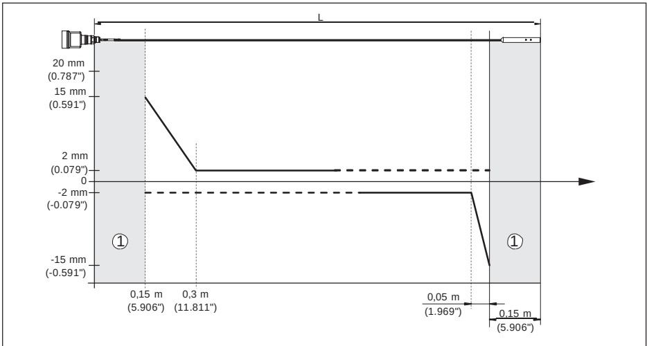
Рис. 52: Погрешность измерения SITRANS LG250 в тросовом исполнении \varnothing 4 мм (0.157 in), продукт - масло
