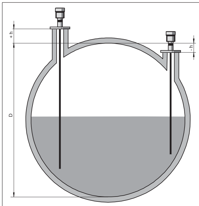
Рис. 30: Высота емкости и значение коррекции патрубка
