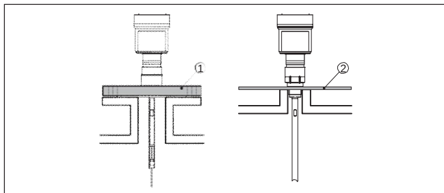
Рис. 1: Монтаж на неметаллической емкости
