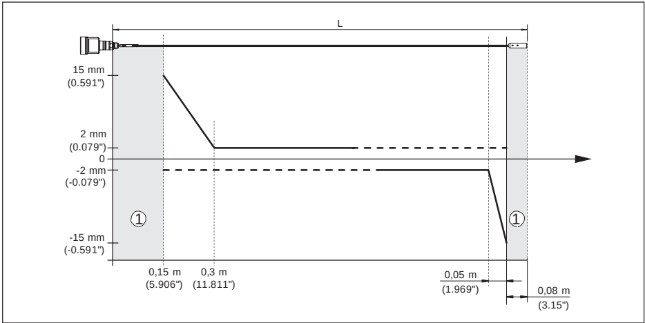
Рис. 51: Погрешность измерения SITRANS LG250 в тросовом исполнении \varnothing 2 мм (0.079 in), продукт - масло
