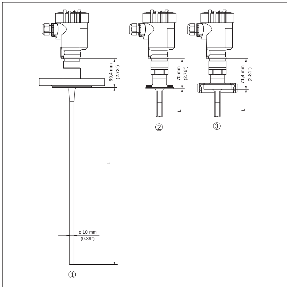
Рис. 55: SITRANS LG240, стержневое исполнение
