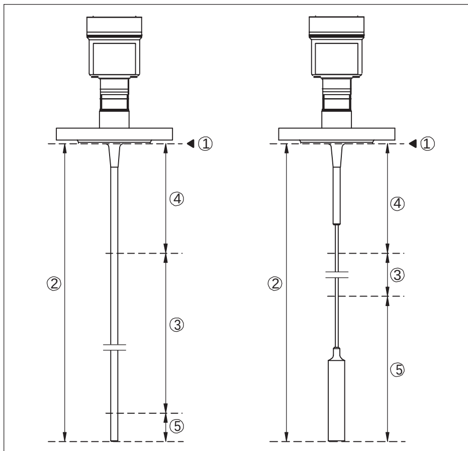
Рис. 43: Диапазоны измерения - SITRANS LG240
