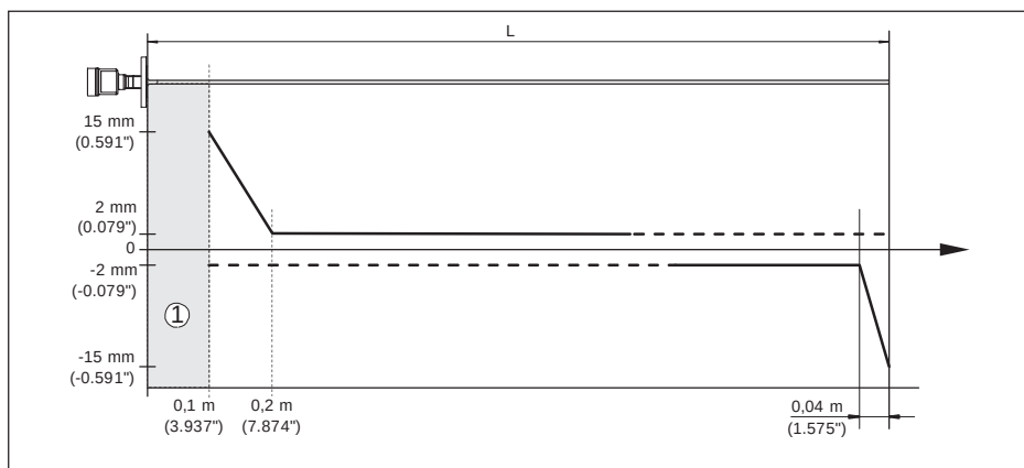
Рис. 44: Погрешность измерения SITRANS LG240 в стержневом исполнении с покрытием (продукт - вода)
