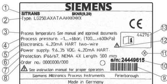
Рис. 4: Данные на типовом шильдике (пример)
