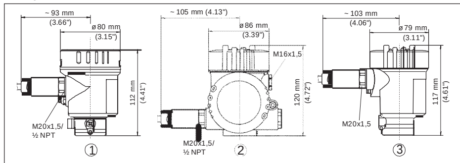
Рис. 53: Корпуса в исполнении IP 66/IP 68 (1 bar) - с установленным модулем индикации и настройки корпус выше на 9 mm/0.35 in
