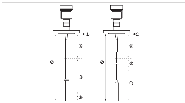
Рис. 3: Диапазоны измерения - SITRANS LG240
