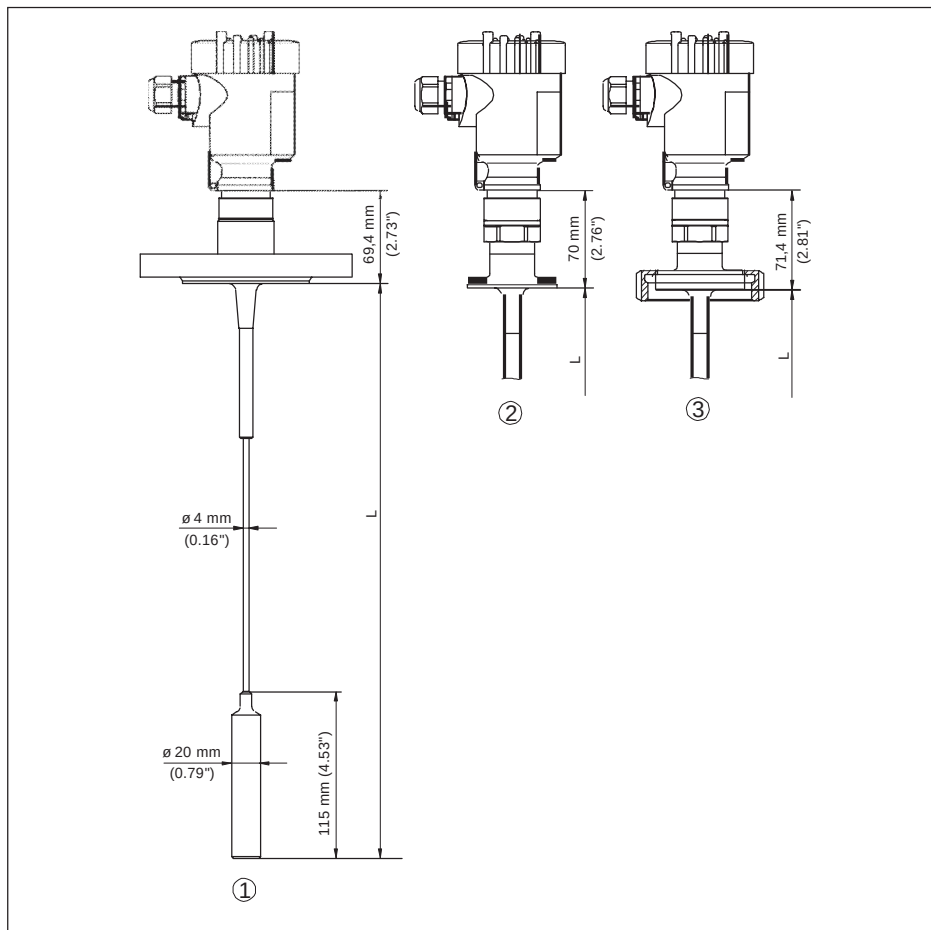
Рис. 54: SITRANS LG240, тросовое исполнение с натяжным грузом
