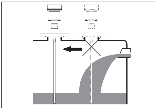
Рис. 11: Монтаж датчика при втекающем продукте
