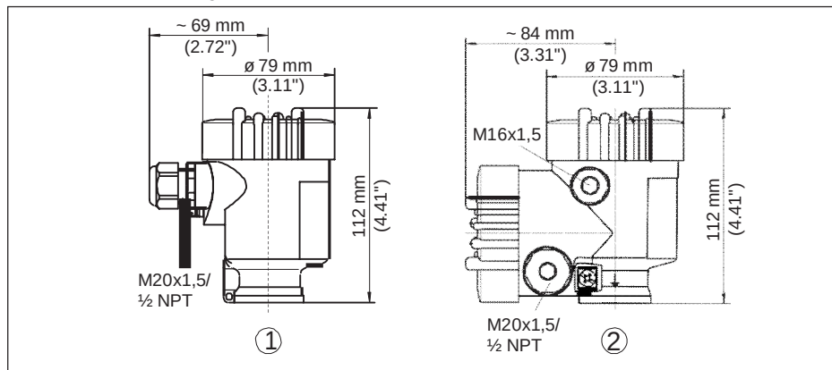
Рис. 49: Корпуса в исполнении IP 66/IP 68 (0,2 bar) - с установленным модулем индикации и настройки корпус выше на 9 мм/0.35 in
