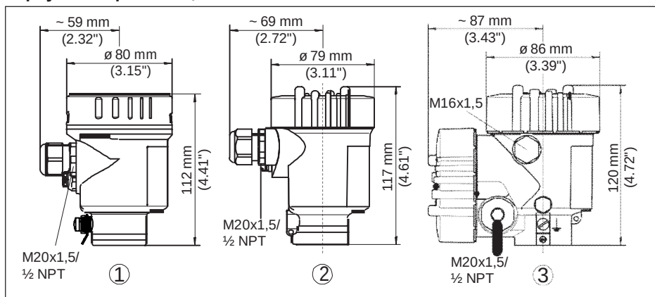
Рис. 52: Корпуса в исполнении IP 66/IP 68 (0,2 bar) - с установленным модулем индикации и настройки корпус выше на 9 мм/0.35 in
