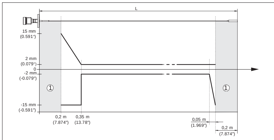
Рис. 47: Погрешность измерения SITRANS LG240 в тросовом исполнении с покрытием (продукт - масло)
