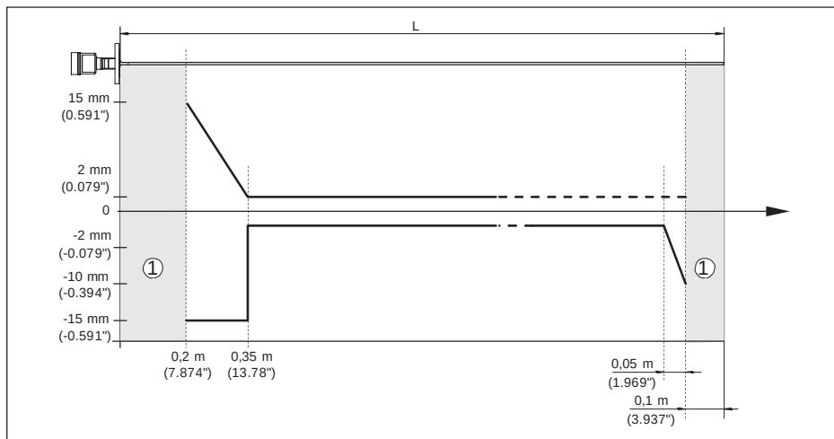
Рис. 45: Погрешность измерения SITRANS LG240 в стержневом исполнении с покрытием (продукт - масло)
