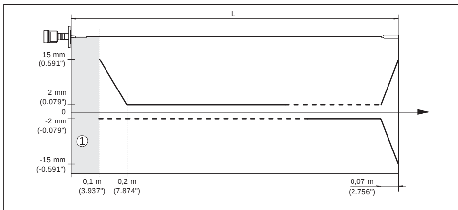
Рис. 46: Погрешность измерения SITRANS LG240 в тросовом исполнении с покрытием (продукт - вода)
