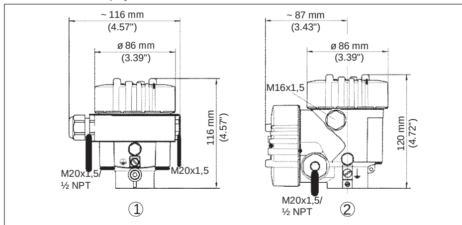
Рис. 50: Корпуса в исполнении IP 66/IP 68 (0,2 bar) - с установленным модулем индикации и настройки корпус выше на 9 мм/0.35 in
