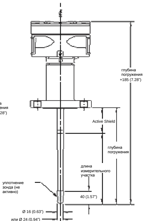
Серия S, обработанный фланец
