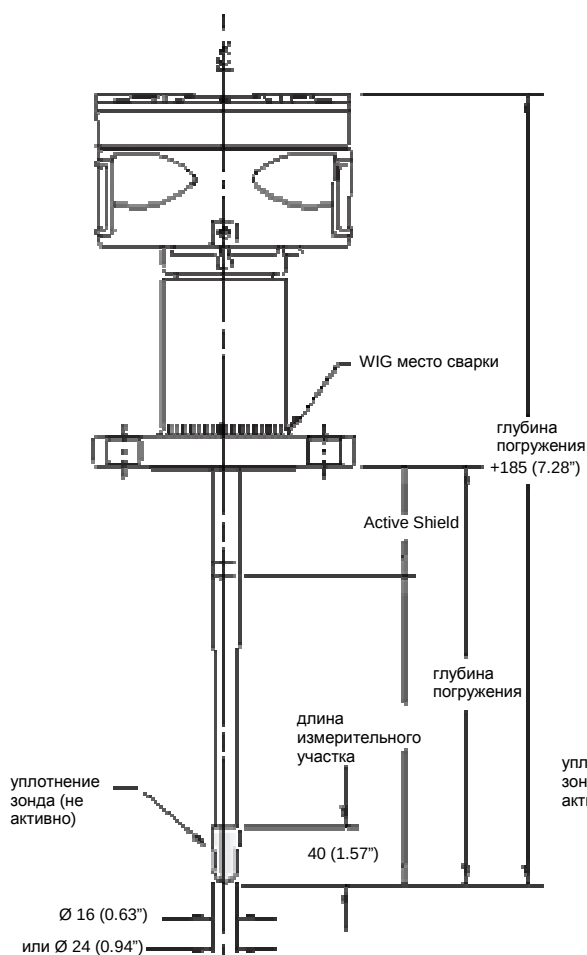
Серия S, сварной фланец
