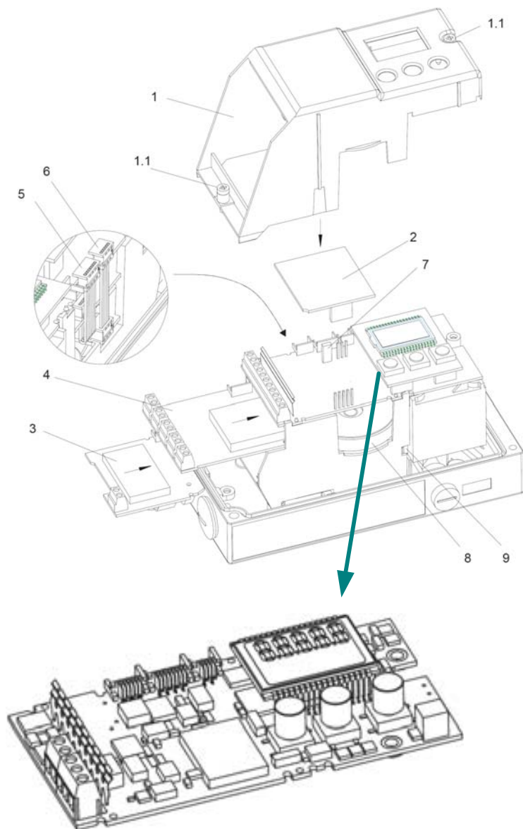
Рисунок 1. Материнская плата
