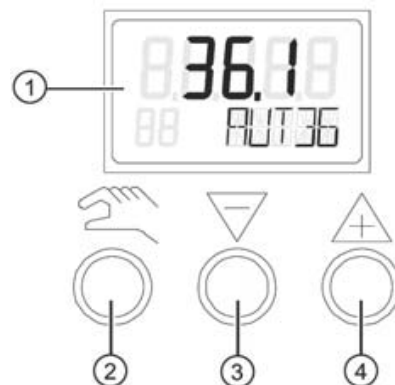
Рисунок.2 Цифровой дисплей и кнопки позиционера
