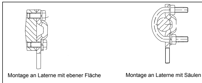
Bild 5 Montagebeispiel für Schubantrieb bis 14 mm
