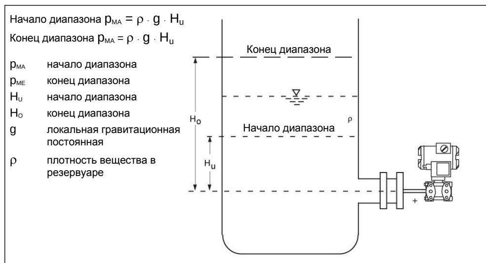
Рис. 25. Измерение уровня в открытом резервуаре
