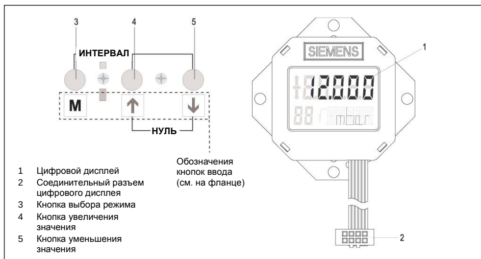
Рис. 20 Расположение клавиатуры (три кнопки ввода)
