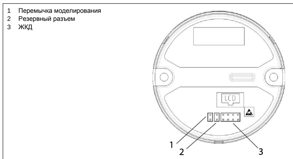
Рис. 21 Разъемы и переключки
