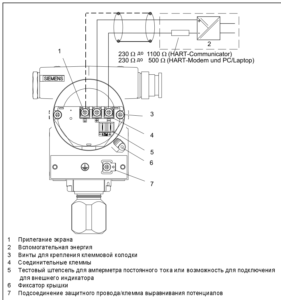
Bild 38 Электрическое подсоединение, схема
