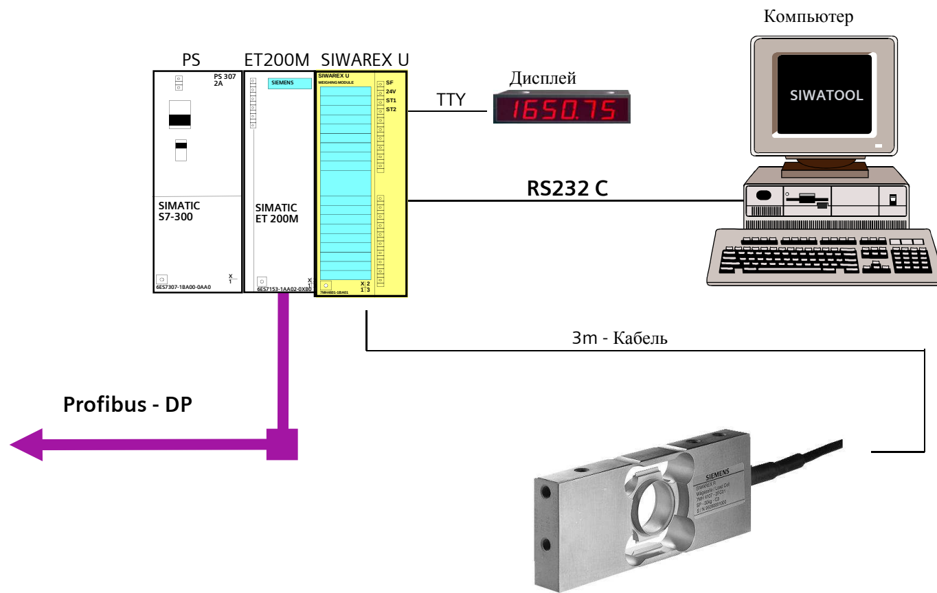
Весовой датчик Type SP , Нагрузка 6kg
