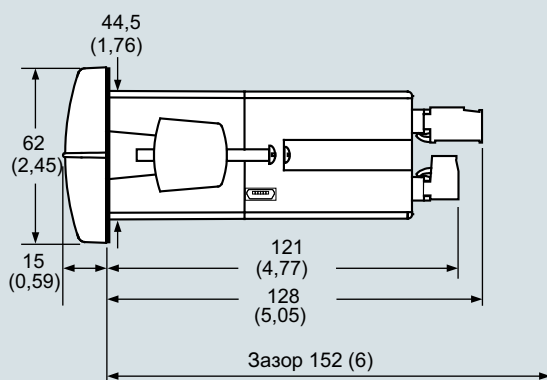
SITRANS RD300, размеры в мм (дюймах)
