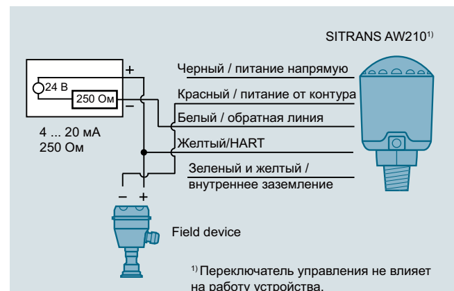
Питание от контура для подключения одного устройства 4...20 мА HART
