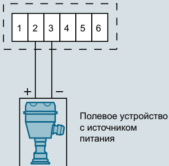
Подключение 4-проводного полевого устройства
