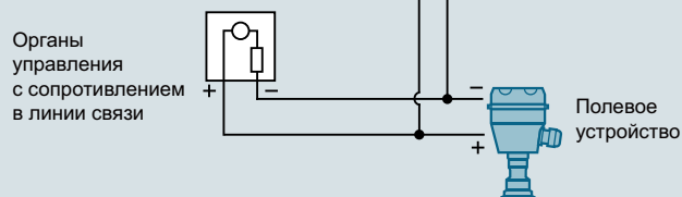
Подключение адаптера параллельно подключенным устройствам обмена данными с интерфейсом 4...20 мА
