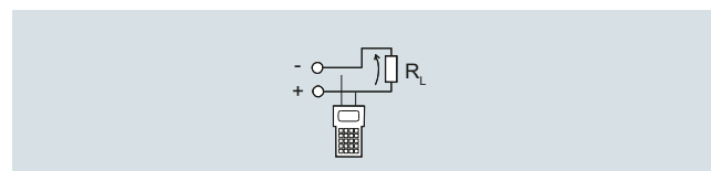
Разделитель питания SITRANS I100 с HART, конфигурация выхода
