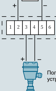
Подключение 2-проводного полевого устройства с внешним источником питания
