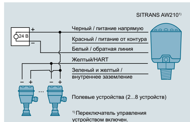
Внешний источник питания 24 В DC, подключение нескольких устройств
