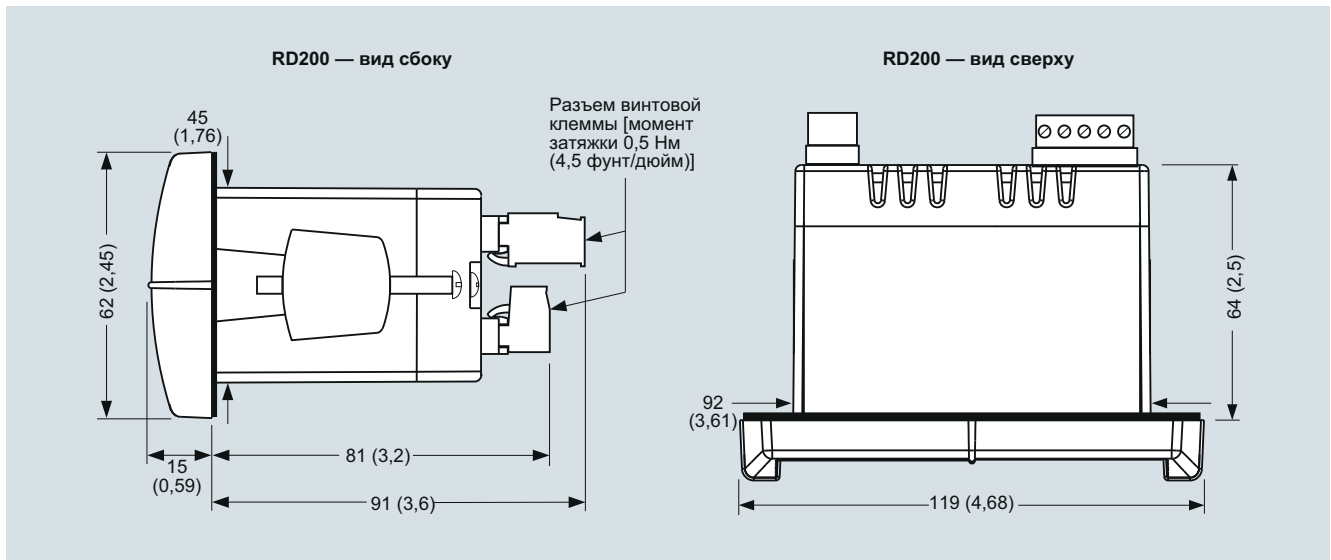
SITRANS RD200, размеры в мм (дюймах)
