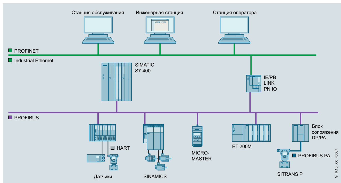
Примерная конфигурация: использование IE/PB LINK PN IO в качестве шлюза по умолчанию без TIA Portal / STEP 7
