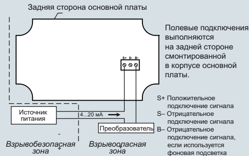
Рис. 2. Контур управления, подключенный к основной плате с фоновой подсветкой
