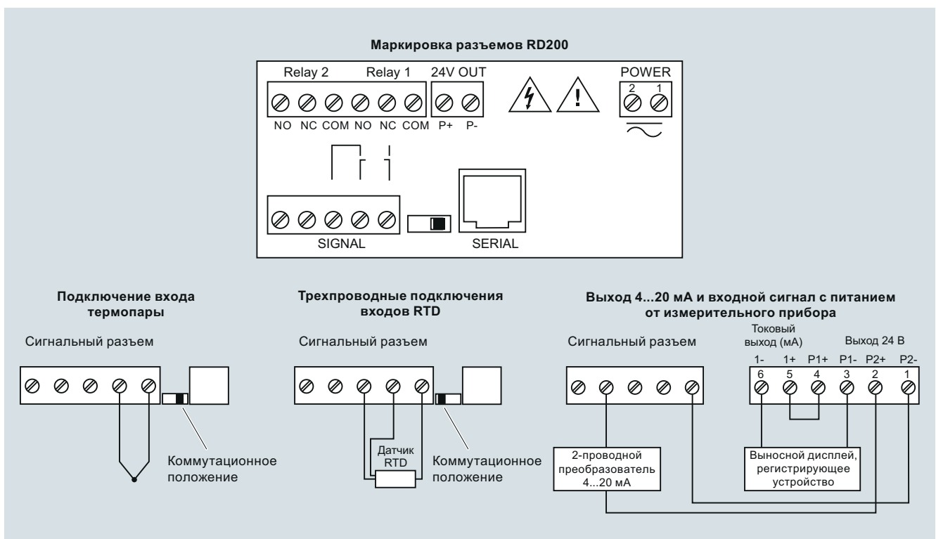
Подключения SITRANS RD200
