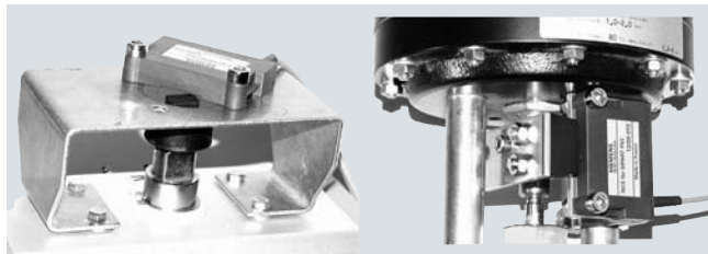
Контактный и бесконтактный датчики положения (NCS) для поворотного привода (слева) и поступательного привода \leq 14 мм (справа)
