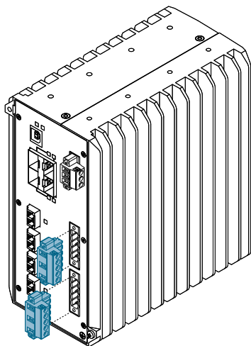
Рисунок 2.8 Сборка клеммных колодок питания
