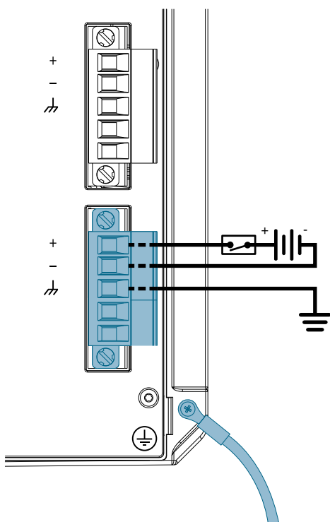
Рисунок 2.15 Схема подключения с одним входом от источника низковольтного питания постоянного тока
