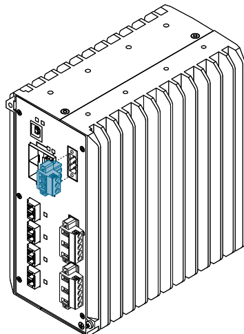
Рисунок 2.6 Сборка клеммной колодки реле аварийной сигнализации
