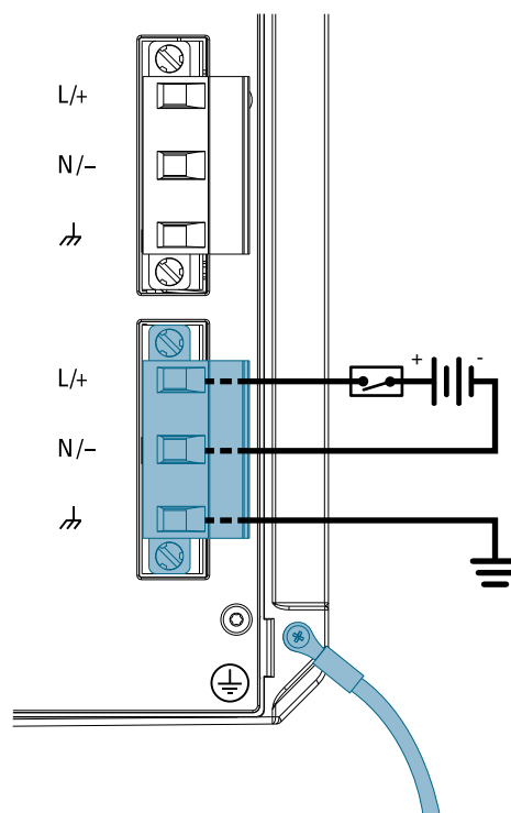
Рисунок 2.12 Схема подключения с одним входом от источника высоковольтного питания постоянного тока
