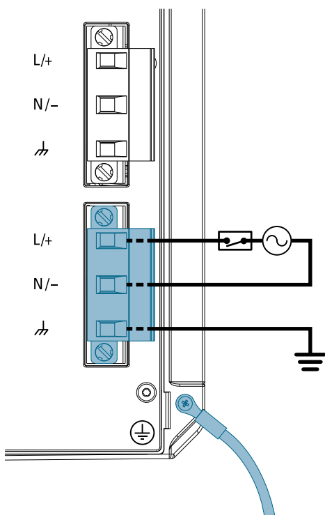
Рисунок 2.11 Схема подключения с одним входом от источника высоковольтного питания переменного тока
