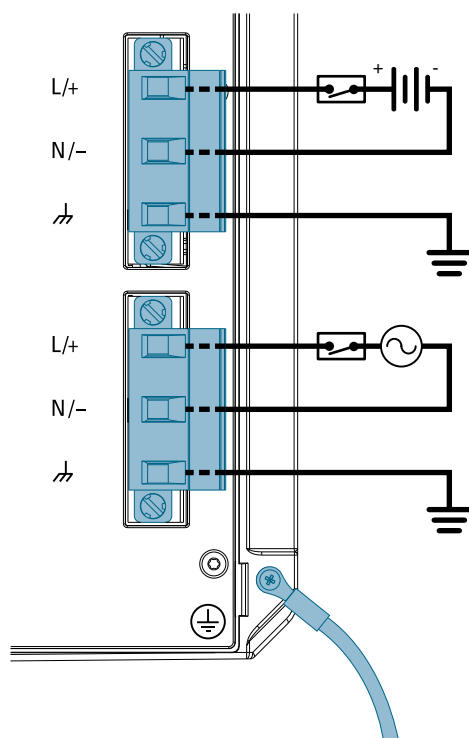
Рисунок 2.13 Два источника высоковольтного питания переменного и постоянного тока
