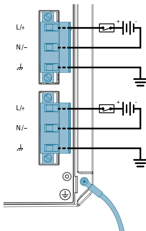
Рисунок 2.14 Два источника высоковольтного питания постоянного тока
