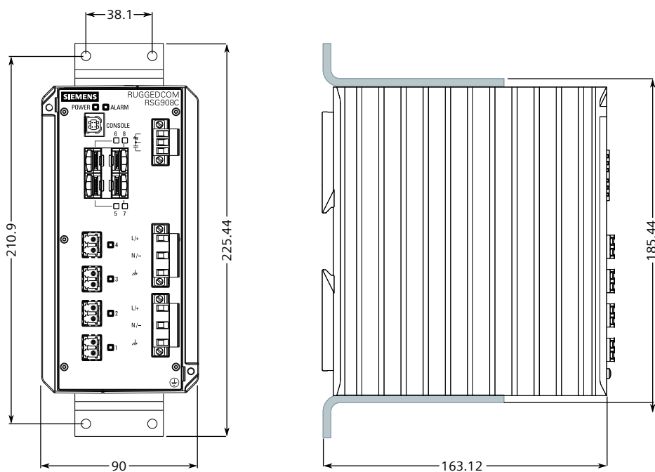
Рисунок 5.2 Размеры при монтаже на панель
