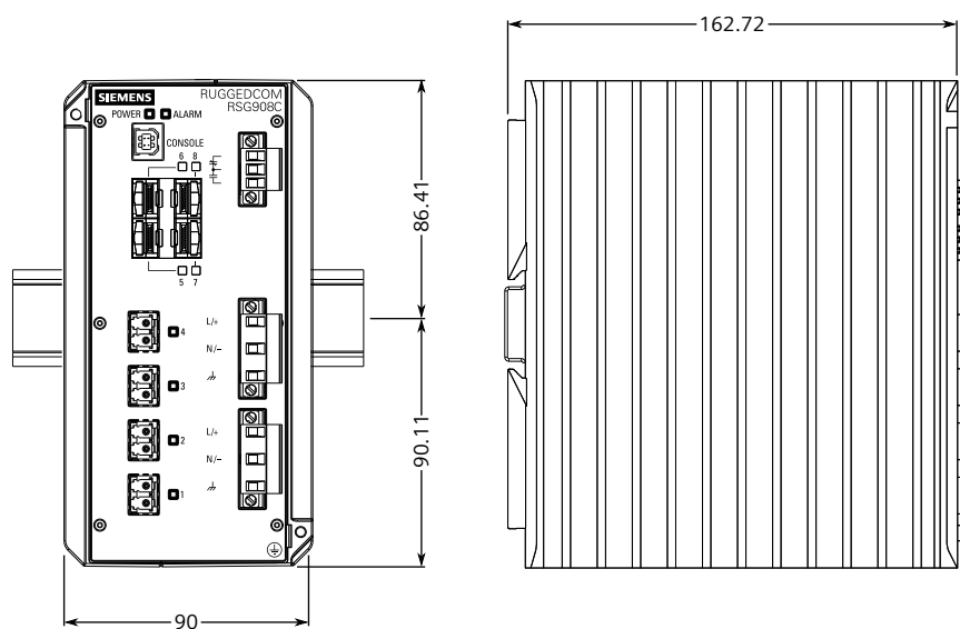
Рисунок 5.3 Размеры при монтаже на DIN-рейку
