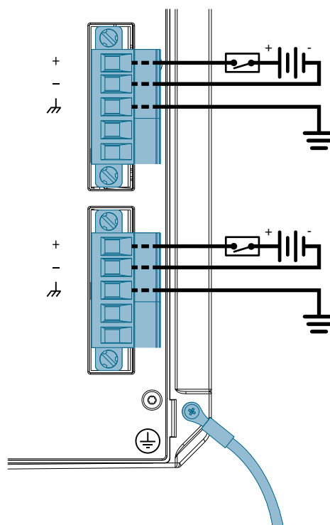
Рисунок 2.16 Схема подключения с двумя входами от источников низковольтного питания постоянного тока
