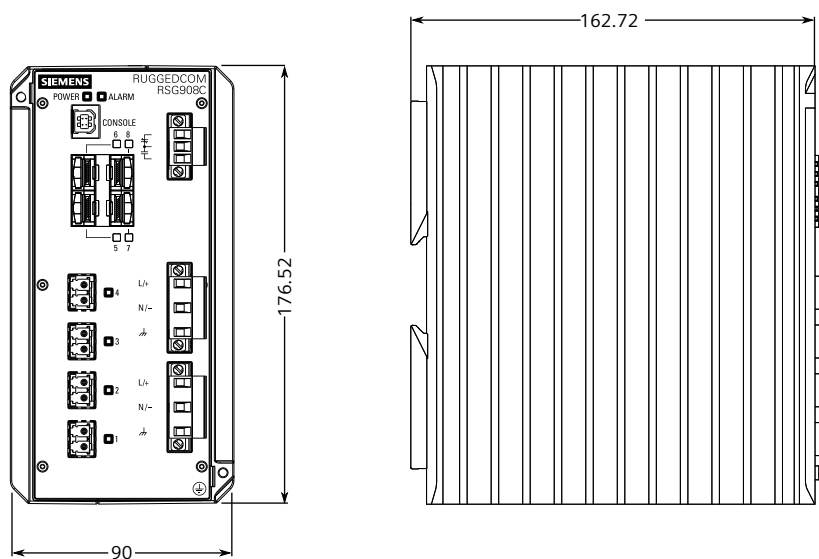
Рисунок 5.1 Габаритные размеры
