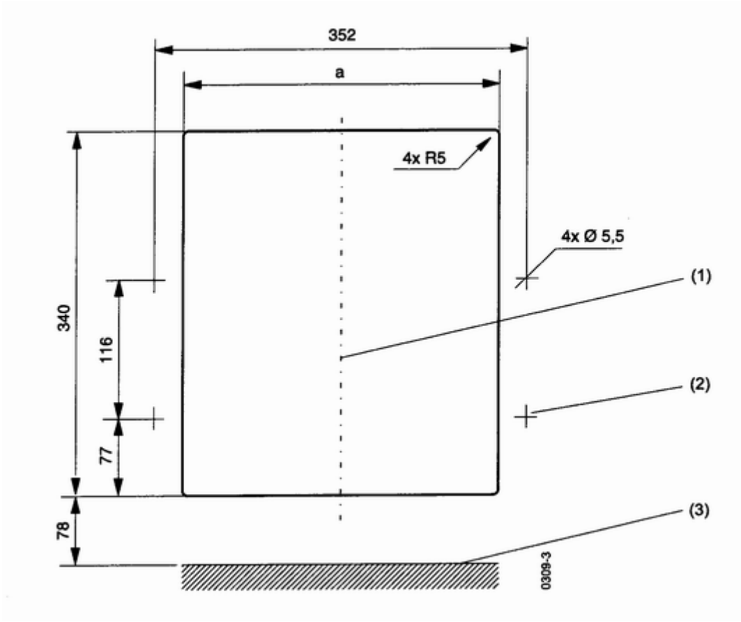
Чертеж с размерами для дверного выреза и установочных отверстий
