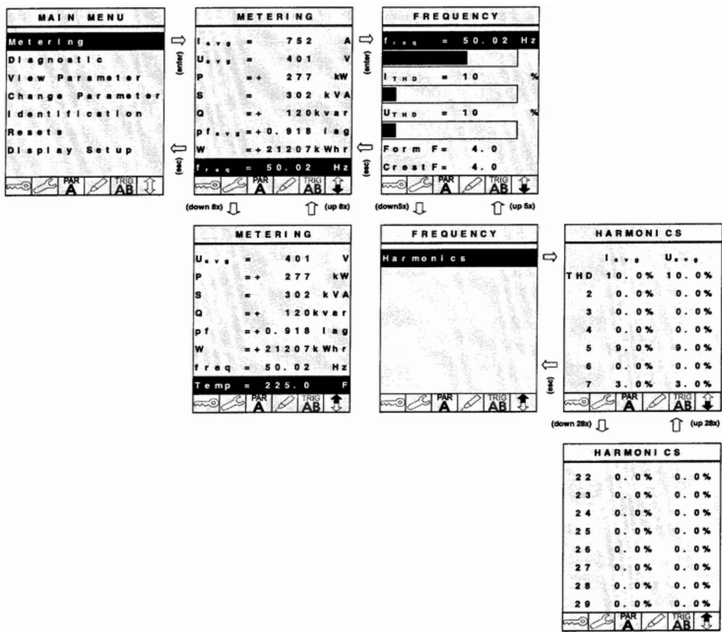
HARMONICS - Гармоники
