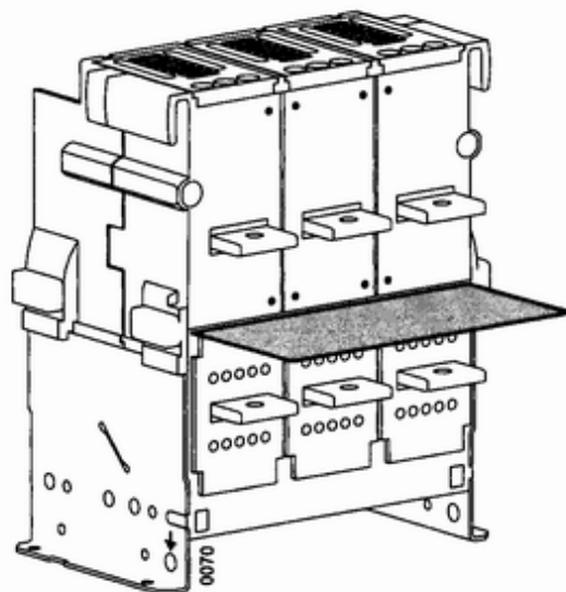
Горизонтальные перегородки
