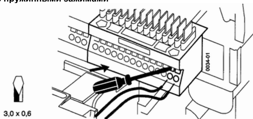
Электрические соединения
