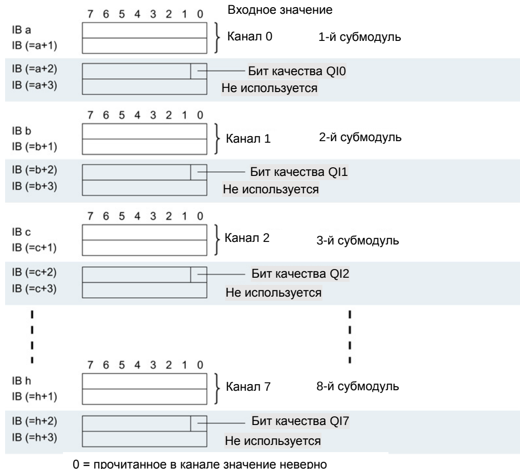
Рисунок 4-3 Адресное пространство для конфигурации 8 x 1 канал AI 8xU/I HS S QI с регистрацией информации о качестве
