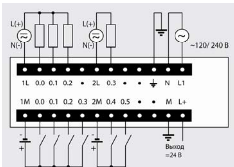
6ES7 211-0BA23-0XB0
