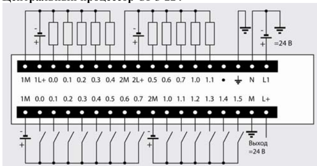
6ES7 214-1AD23-0XB0
