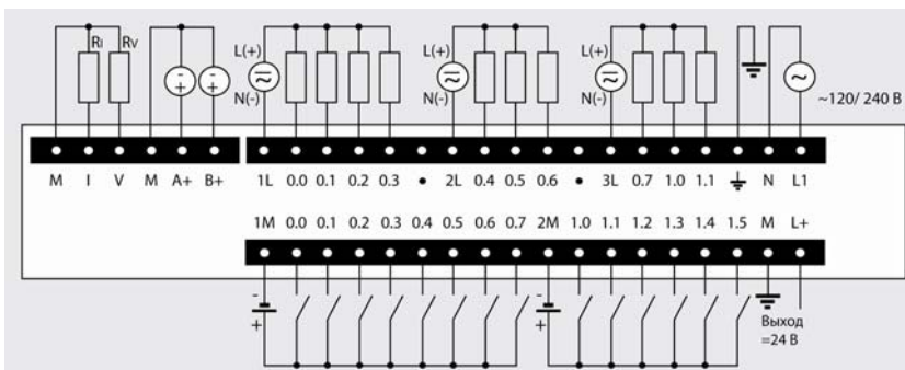
6ES7 224-2BD23-0XB0
