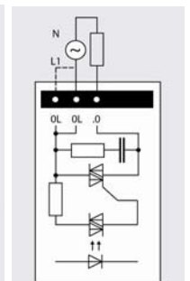
Выход ~120/230 В/ 0.5А
