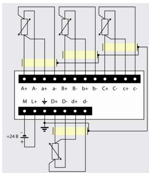
6ES7 231-7PC22-0XA0
