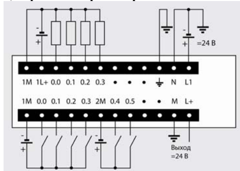
6ES7 211-0AA23-0XB0
