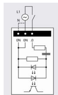
Входные каскады
