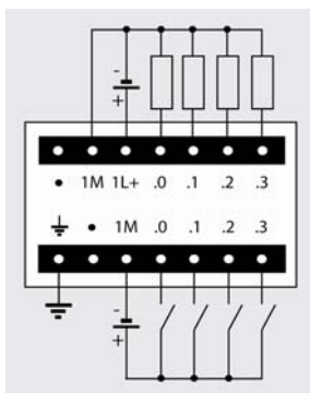
6ES7 223-1BF22-0XA0
