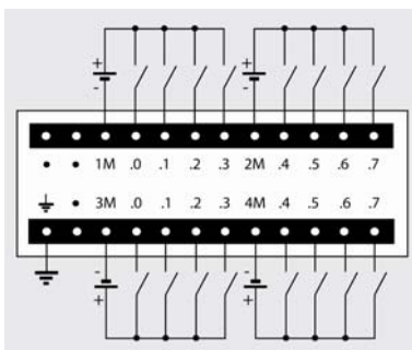
6ES7 221-1BH22-0XA0
