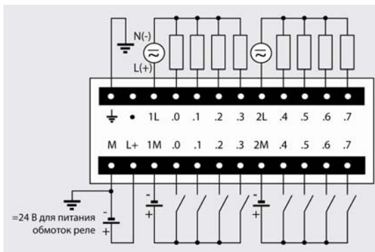
6ES7 223-1PH22-0XA0
