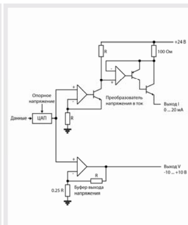
Выходные каскады
