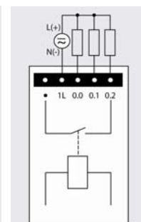
Релейный выход
