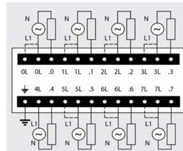
6ES7 222-1EF22-0XA0
