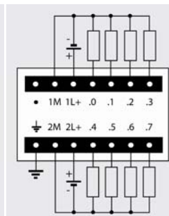
6ES7 222-1BF22-0XA0
