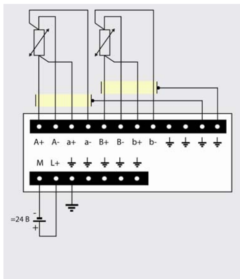
6ES7 231-7PB22-0XA0
