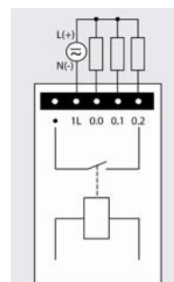
Дискретные выходы с контактами реле
