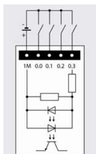
Дискретные входы =24 В
