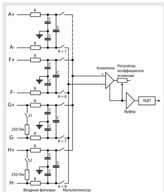
6ES7 231-0HF22-0XA0
