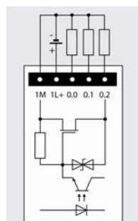
Дискретные выходы =24 В/0.75 А
