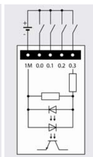
Входные каскады =24 В
