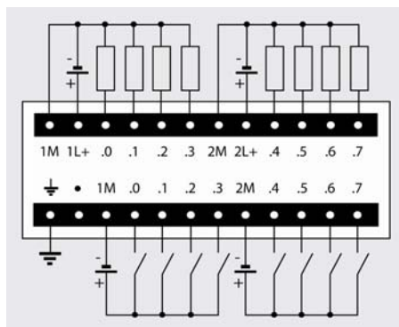
6ES7 223-1BH22-0XA0
