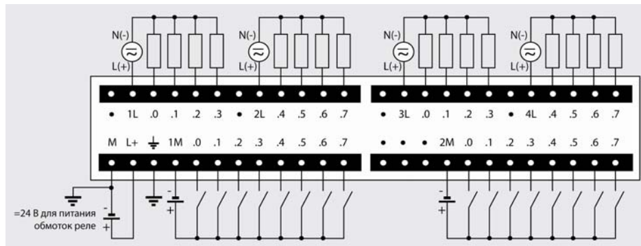
6ES7 223-1PL22-0XA0
