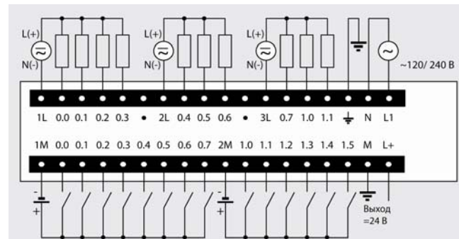
6ES7 214-1BD23-0XB0
