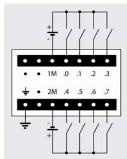
6ES7 221-1BF22-0XA0
