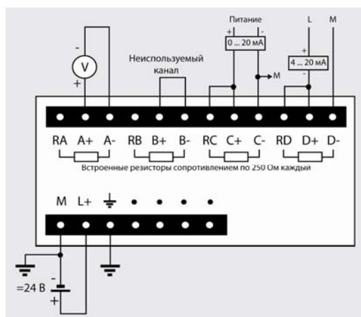
6ES7 231-0HC22-0XA0
