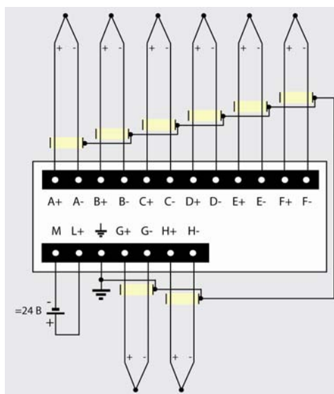
6ES7 231-7PF22-0XA0
