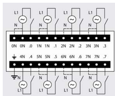
6ES7 221-1EF22-0XA0
