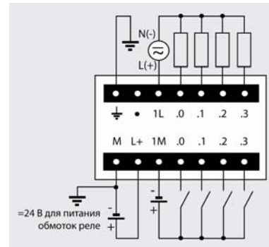
6ES7 223-1HF22-0XA0
