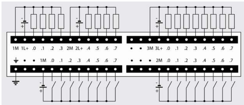
6ES7 223-1BL22-0XA0
