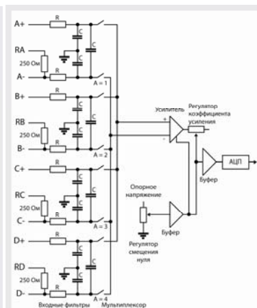
Входные каскады
