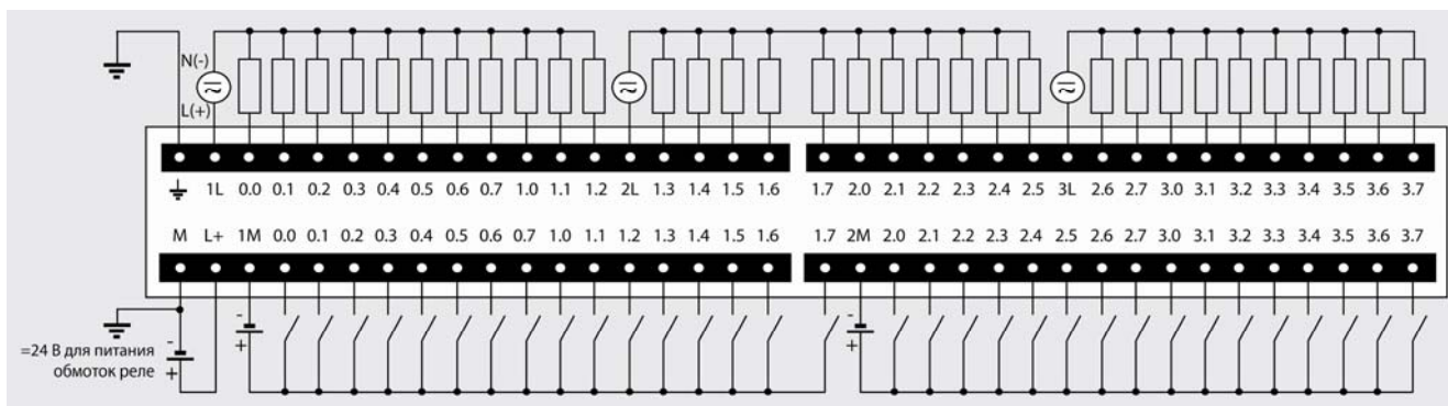
6ES7 223-1PM22-0XA0
