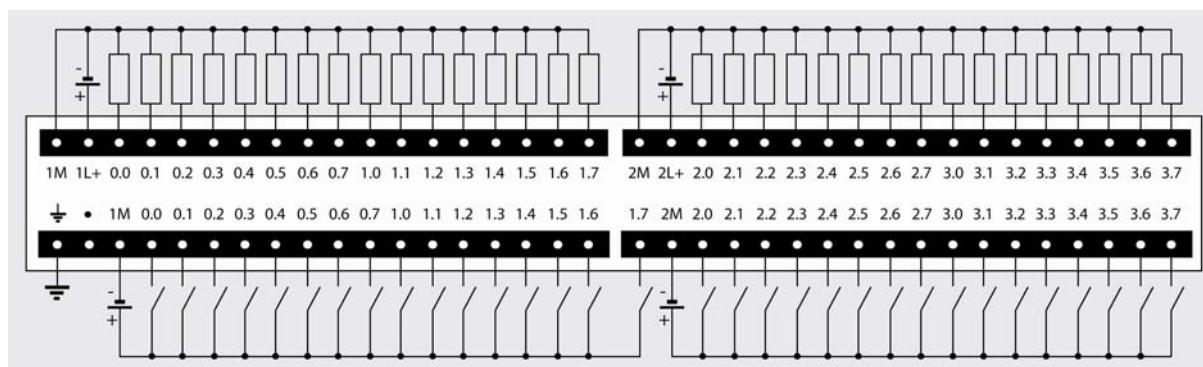
6ES7 223-1BM22-0XA0
