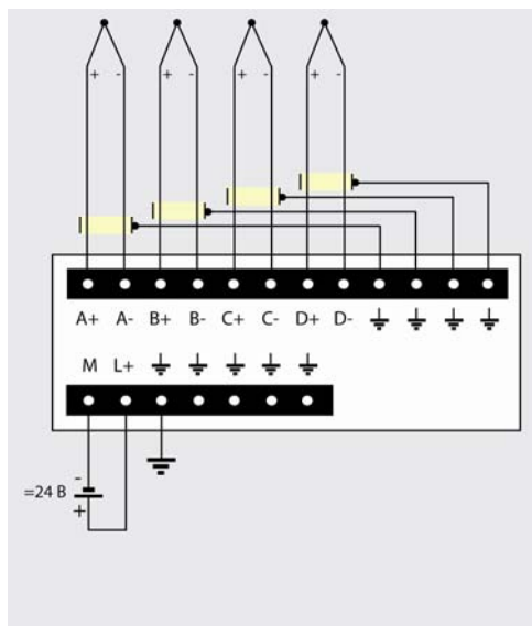
6ES7 231-7PD22-0XA0
