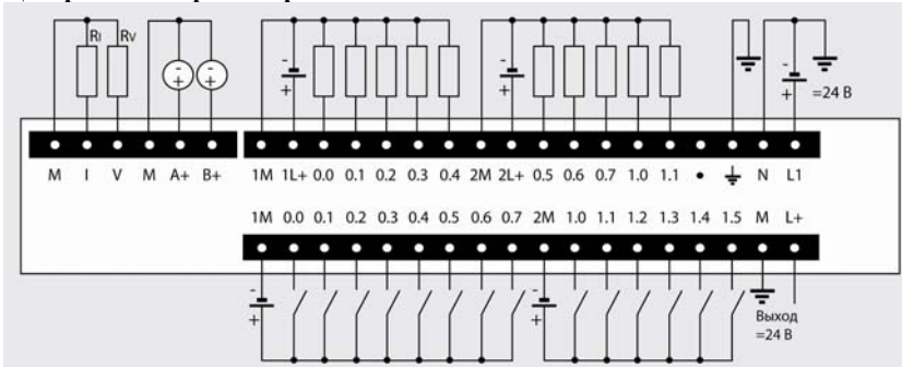
6ES7 214-2AD23-0XB0
