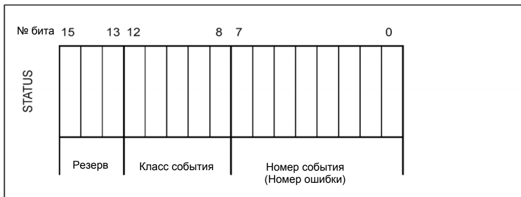
Рис. 8.1 Структура параметра STATUS
