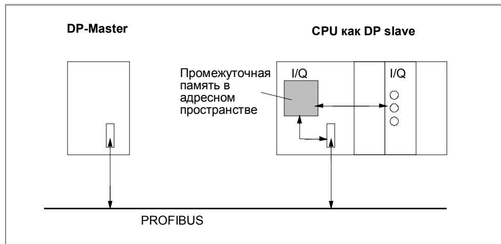
Рис. 9-10. Промежуточная память в CPU 31x-2 DP/31xC-2 DP, используемом как DP-Slave
