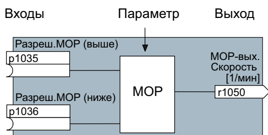
Изображени Пример блока: Моторпотенциометр (МОР) е А-5
