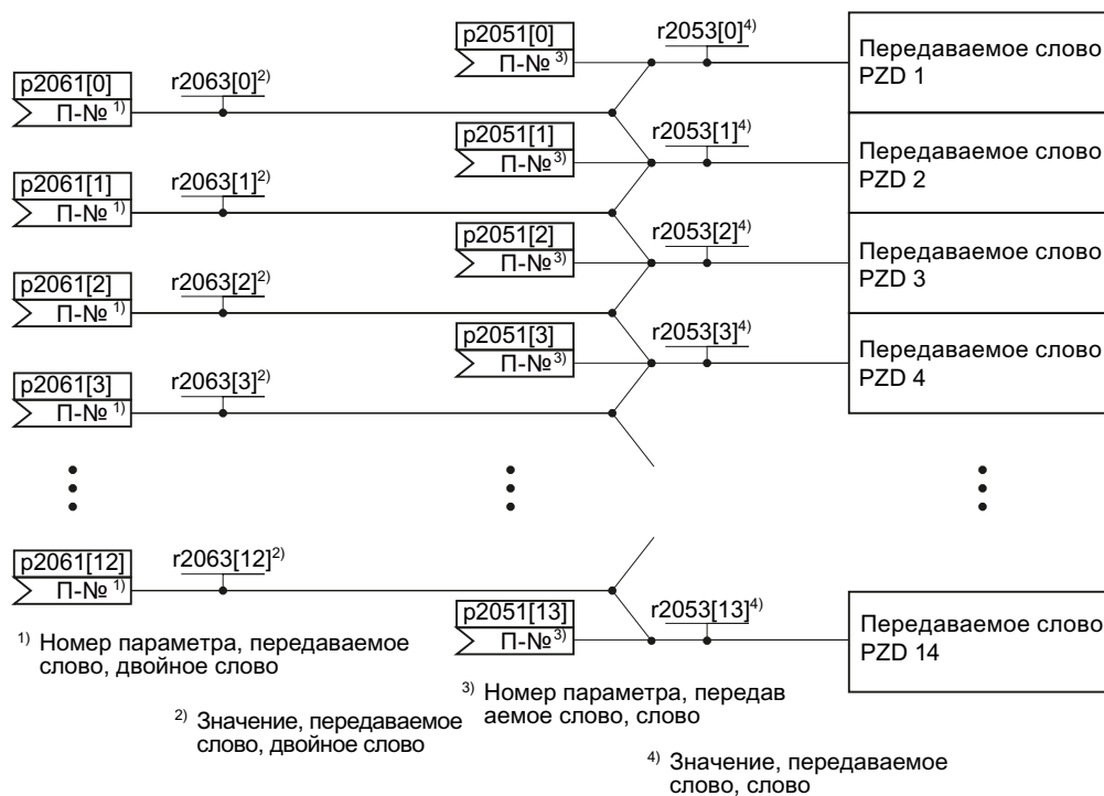
Изображены Подключение передаваемых слов е 7-3
