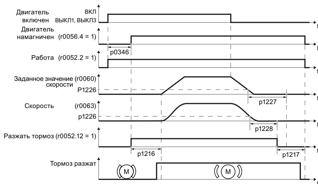
Изображены Управление стояночным тормозом двигателя при включении и выключении е 8-27 двигателя
