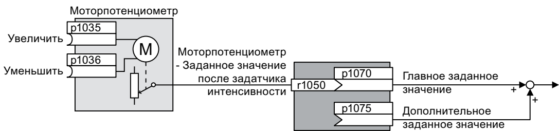
Изображени Моторпотенциометр как источник заданного значения е 8-14
