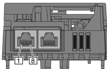
Разъем RJ45 для PROFINET IO (X150 P1, X150 P2)
