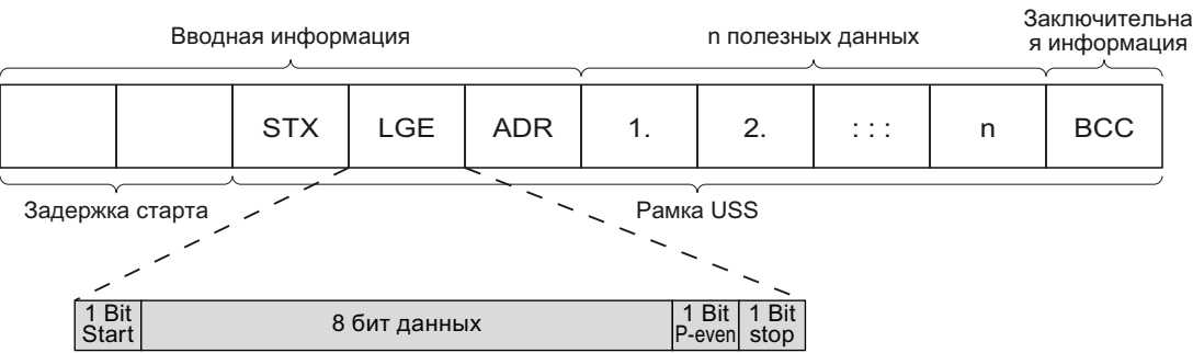
Изображени Структура телеграммы USS е 7-9
