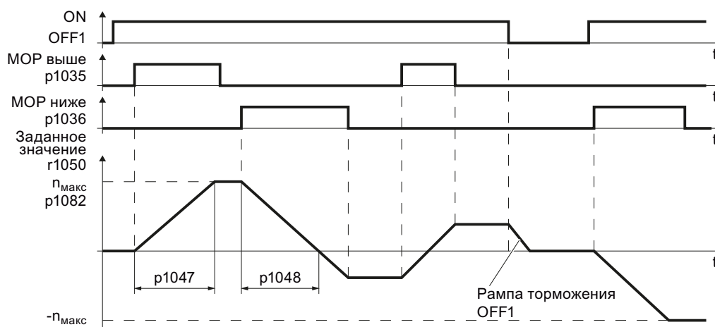
Изображени Функциональная схема моторпотенциометра е 8-15
