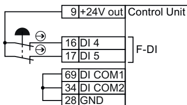
Изображени Подключение чувствительного элемента, к примеру, грибового выключателя е A-14 аварийного останова или концевого выключателя
