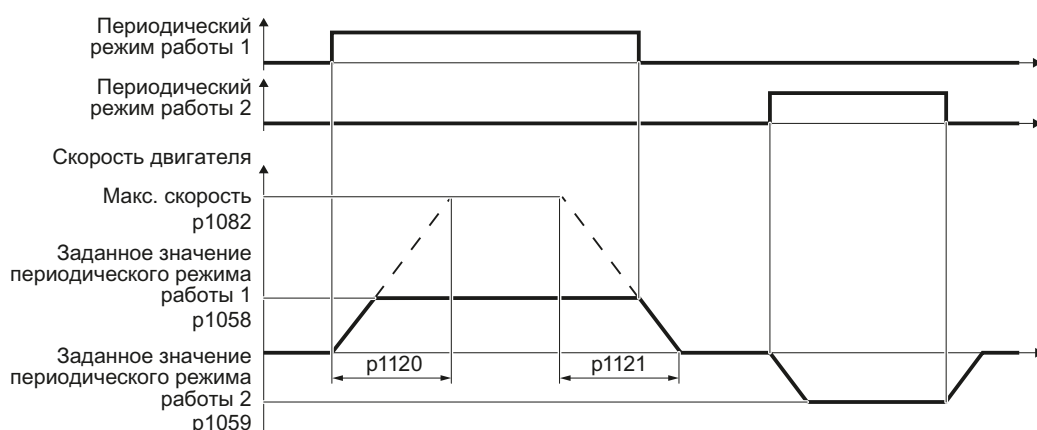
Изображени е 8-8 Поведение двигателя в "Периодическом режиме работы"
