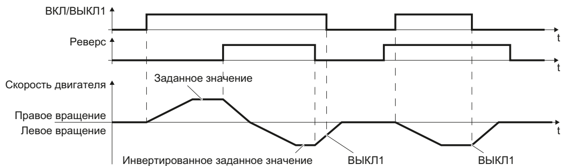
Изображени Двухпроводное управление, метод 1 е 8-3
