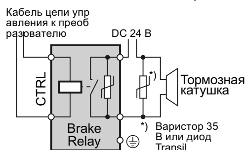
Подключение тормоза 24 В
