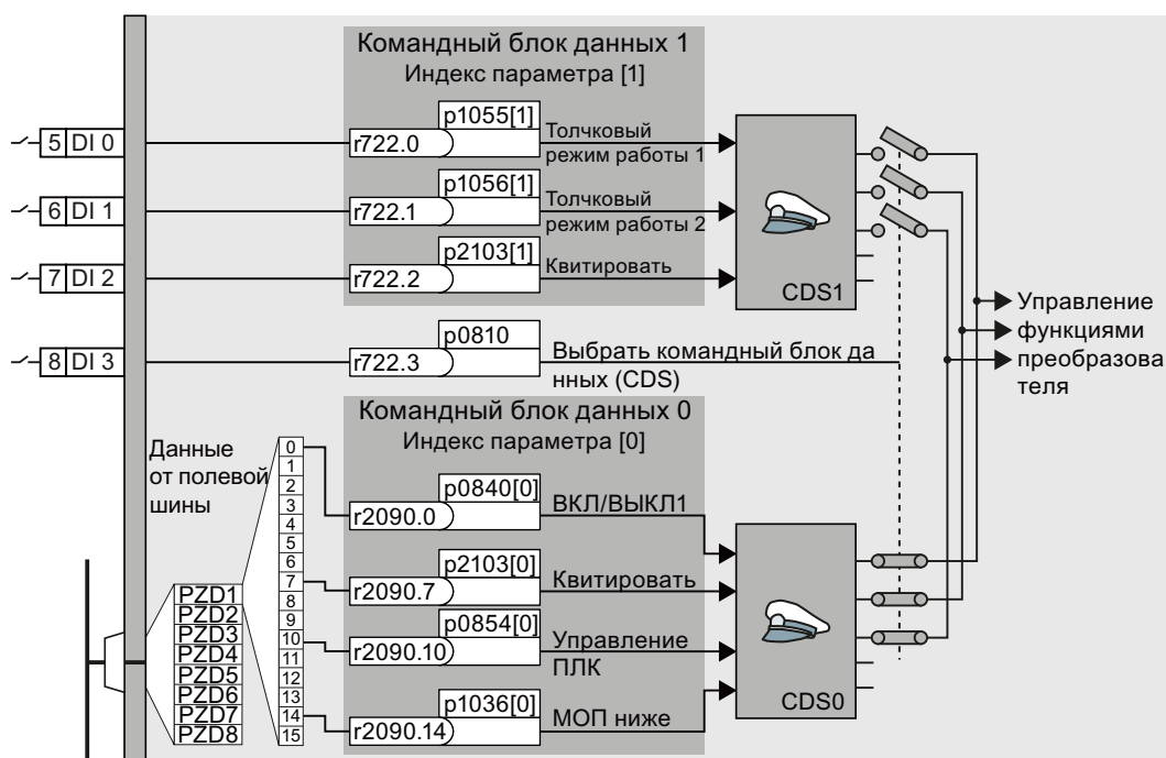
Изображени е 8-10 Пример: Переключение с управления через клеммную колодку на управление по PROFIBUS или PROFINET
