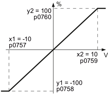
Изображени Примеры нормирующих характеристик е 6-3
