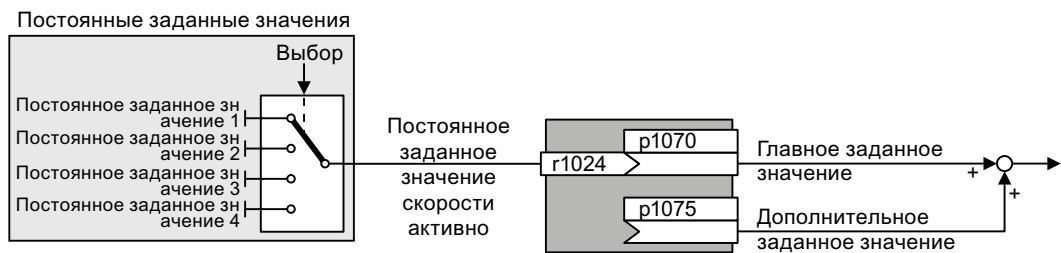
Изображени Постоянные скорости как источник заданного значения е 8-16
