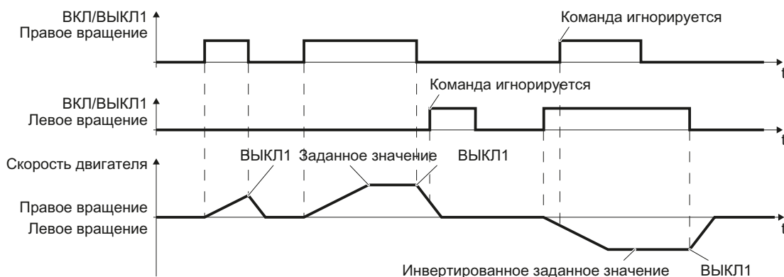
Изображени Двухпроводное управление, метод 2 е 8-4
