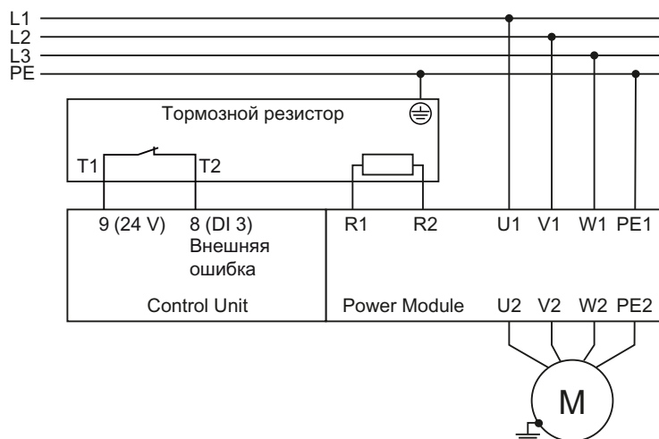
Изображени е 8-25 Подключение тормозного резистора (как пример: контроль температуры через цифровой вход DI 3)
