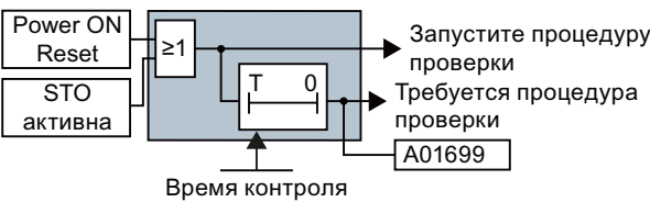
Изображение 8-39 Запуск и контроль процедуры проверки
