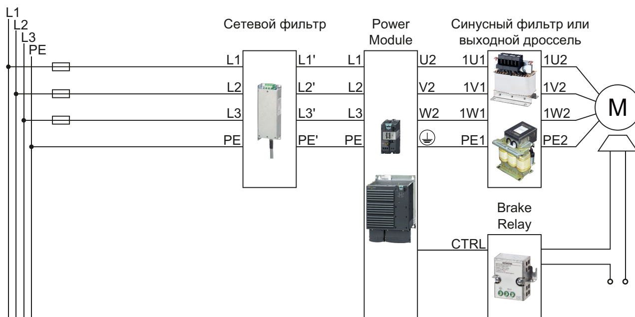
Изображены Подключение силовых модулей PM250 е 4-4
