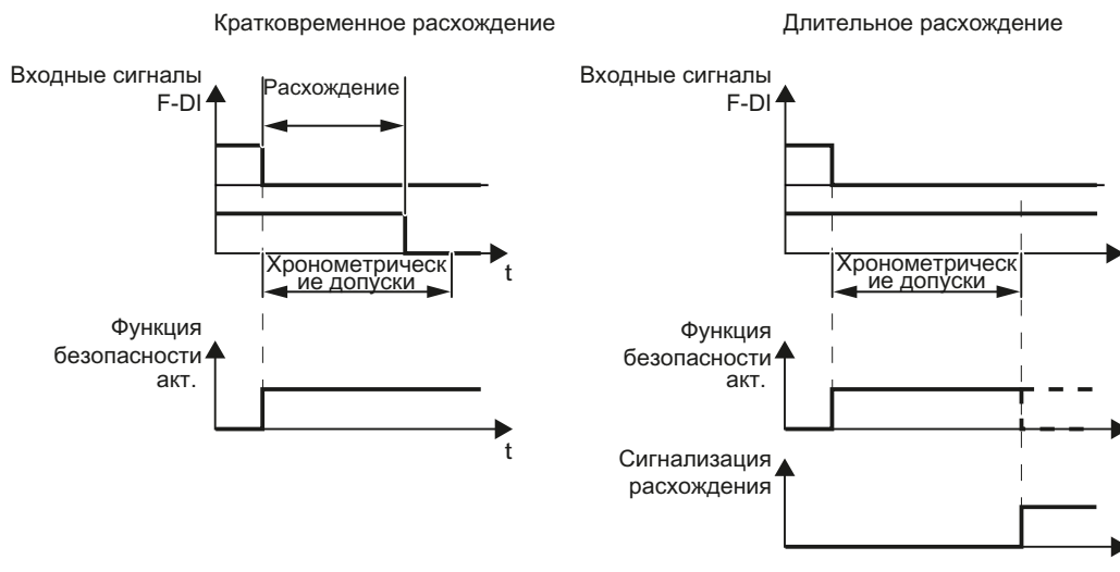
Изображены Допуск для расхождения е 8-36
