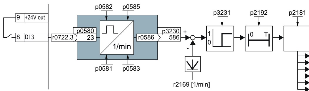
Изображены Контроль на предмет отклонения скорости вращения е 8-35
