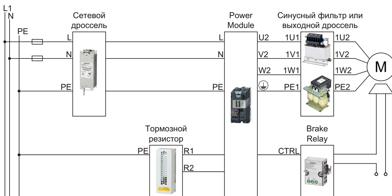
Изображены Подключение силовых модулей PM340 1AC е 4-6
