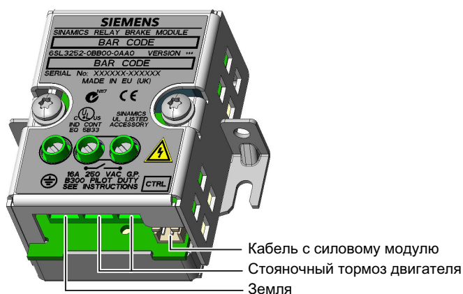
Изображены Соединения реле тормоза е 8-26
