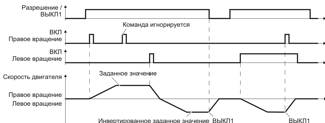
Изображени Трехпроводное управление, метод 1 е 8-6
