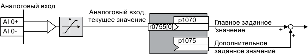
Изображени Пример: Аналоговый вход 0 как источник заданного значения е 8-12
