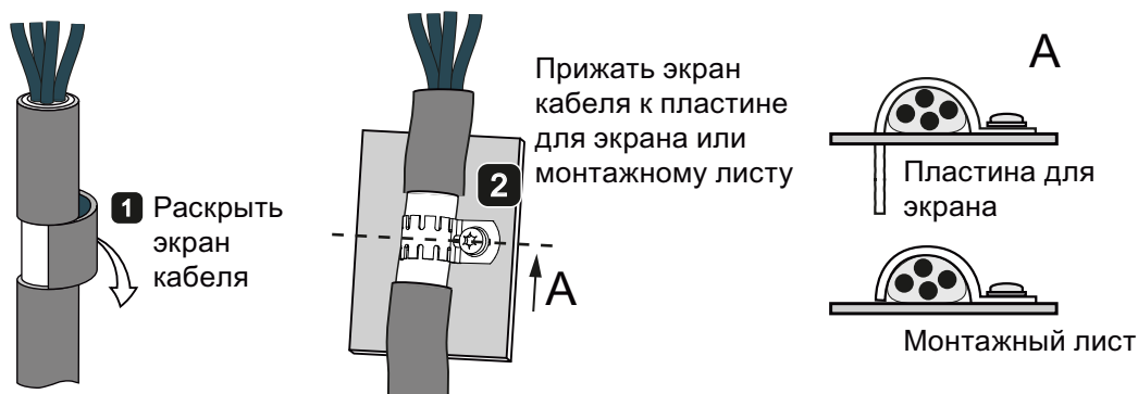
Изображены Заземление экрана - Подробности е 4-10
