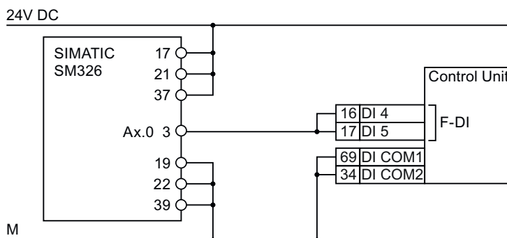
Изображени Подключение F-модуля цифрового вывода, к примеру, SIMATIC F-модуля цифрового е A-16 вывода
