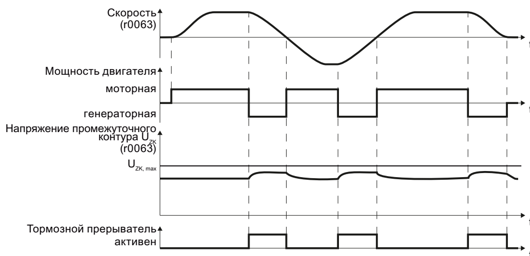
Изображени Упрощенное представление реостатного торможения во времени е 8-24
