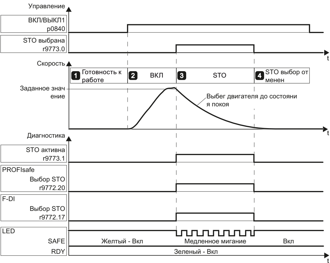
Изображены Приёмочное испытание для STO (базовые функции) е 8-42
