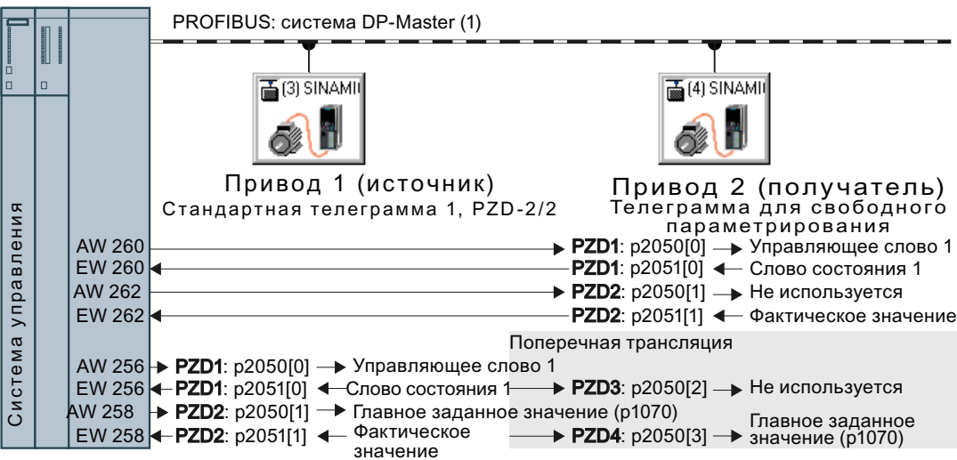
Изображени Коммуникация с контроллером верхнего уровня и между приводами через прямой обмен данными е A-13
