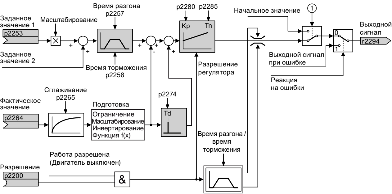
Изображени Упрощенное представление технологического регулятора е 8-32
