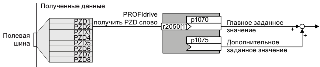
Изображени Полевая шина как источник заданного значения е 8-13
