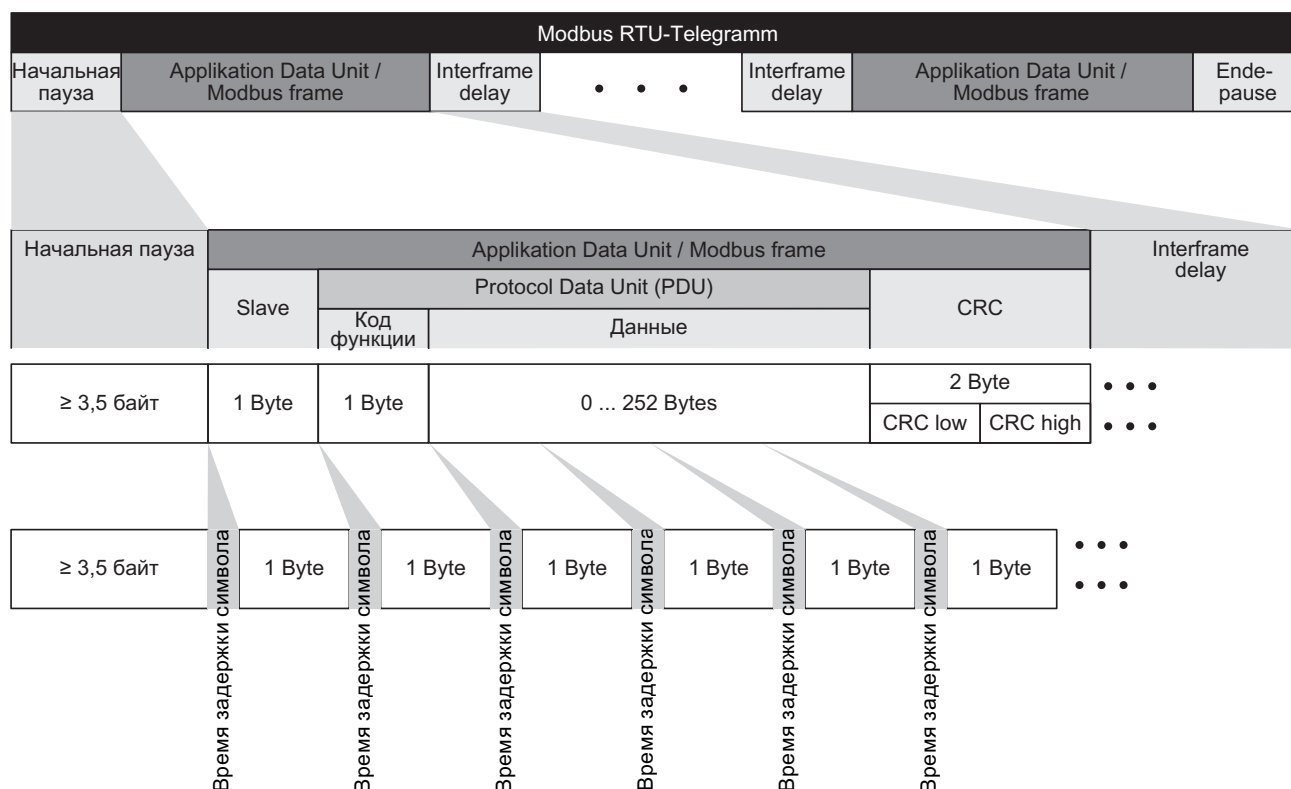
Изображены Modbus с временем задержки е 7-17
