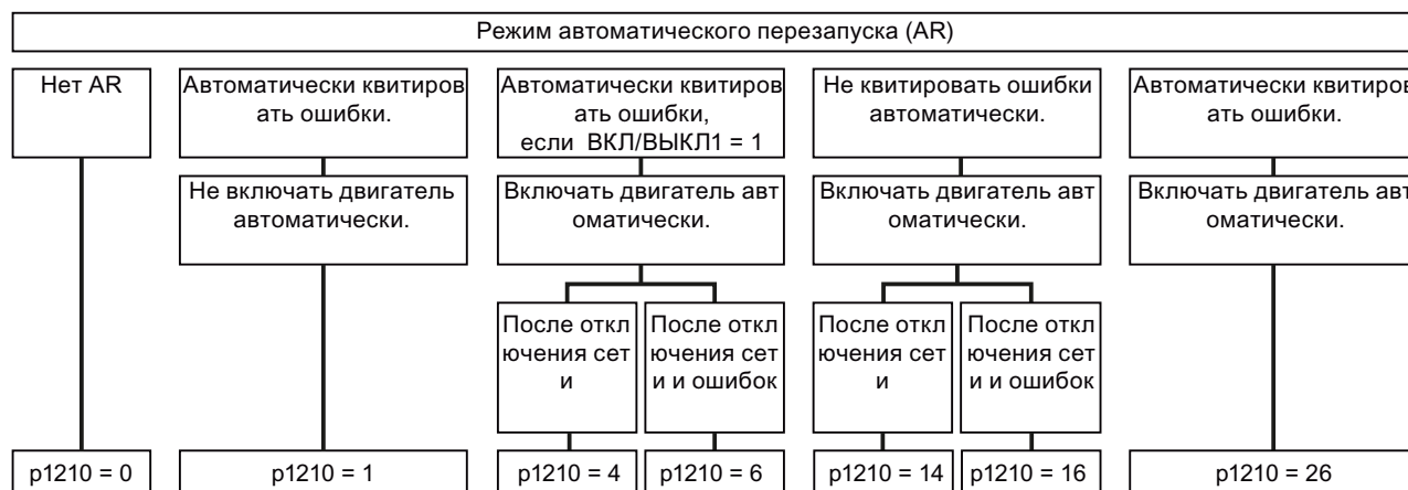
Изображение 8-29 Выбор режима автоматического перезапуска
