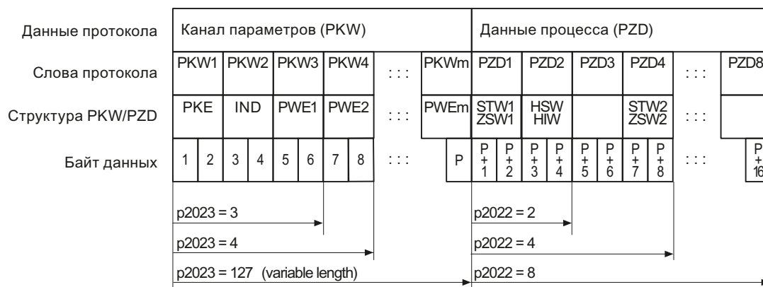
Изображени Телеграмма USS - структура полезных данных е 7-10
