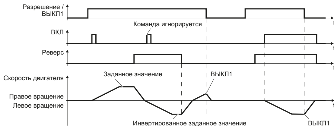
Изображени е 8-7 Трехпроводное управление, метод 2
