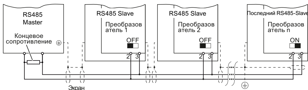
Изображены Коммуникационная сеть через RS485 е 7-8
