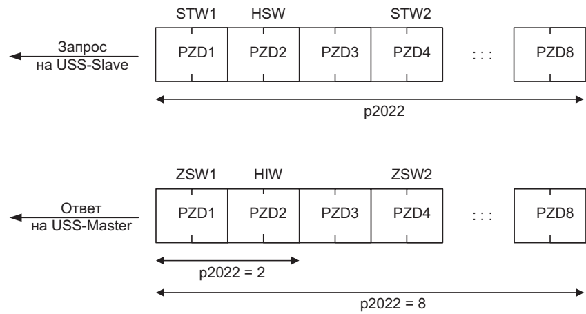
Изображены Канал данных процесса е 7-14
