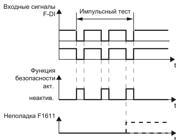
Изображени Реакция преобразователя на импульсный тест е 8-37
