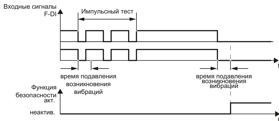
Изображени Фильтр для подавления короткого переключения сигнала е 8-38
