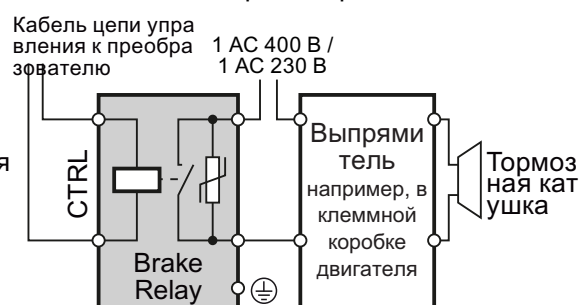
Подключение тормоза 440 В
