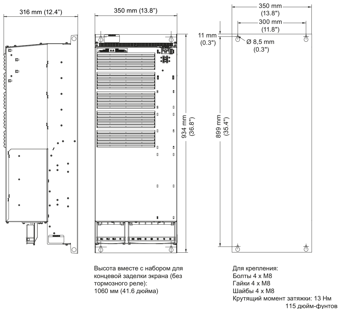
Изображение 3-8 Размеры и сетка отверстий при сверлении, FSF с фильтрацией (НО 45 кВт ... 75 кВт)
