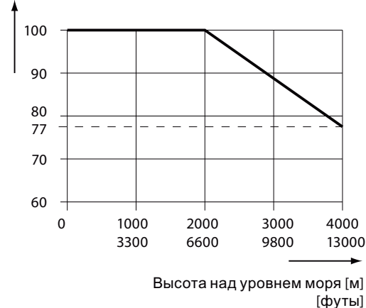
Уменьшение тока в зависимости от высоты Уменьшение напряжения в зависимости от высоты
