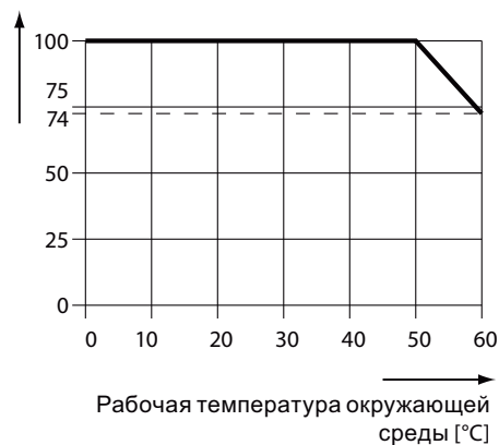
Изображение 6-1 Уменьшение тока в зависимости от температуры
