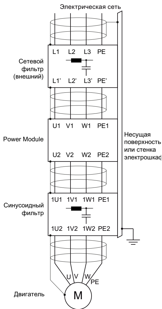
Подключение силовых элементов к синусоидному фильтру
