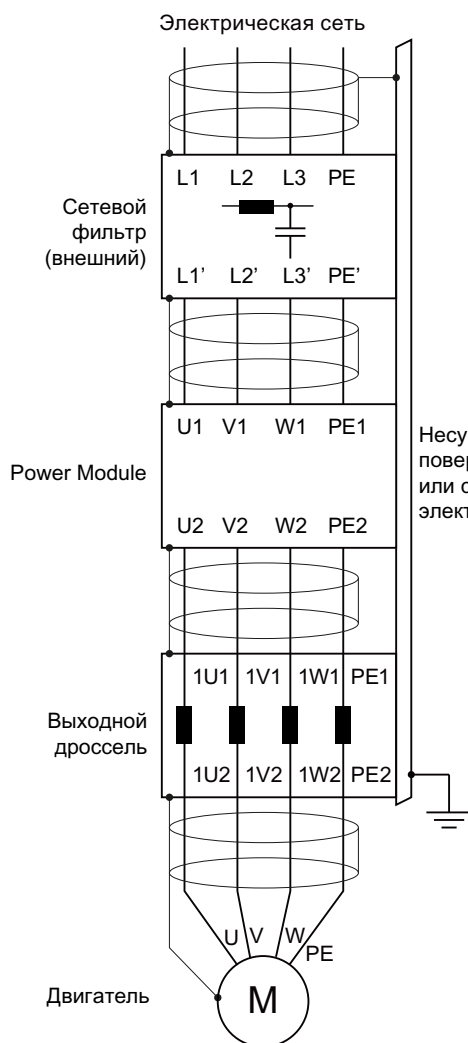
Подключение силовых элементов к выходному дросселю
