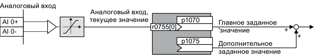
Изображени Пример: Аналоговый вход 0 как источник заданного значения е 8-8
