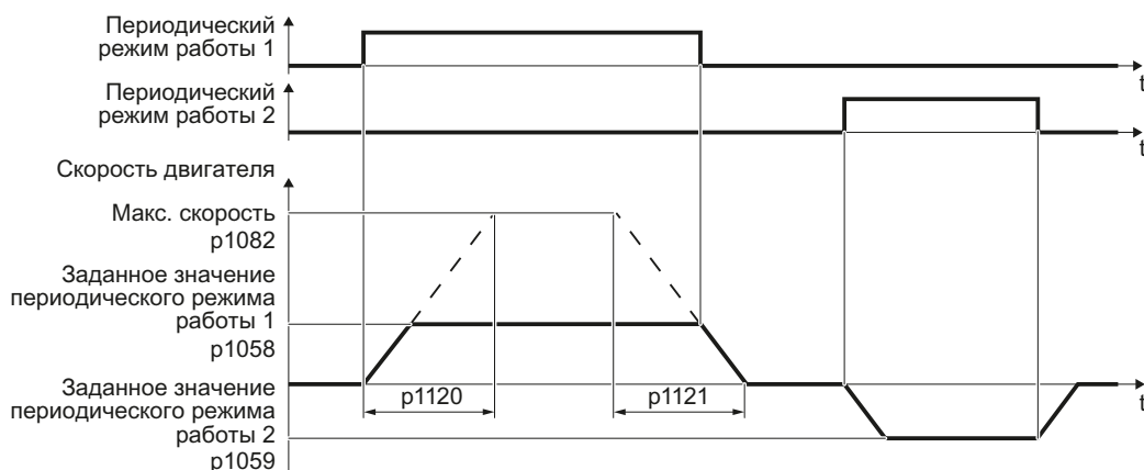
Изображени Поведение двигателя в "Периодическом режиме работы" е 8-3
