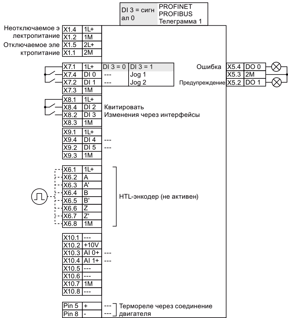
Изображены Подключение согласно заводской установке привода е 5-2
