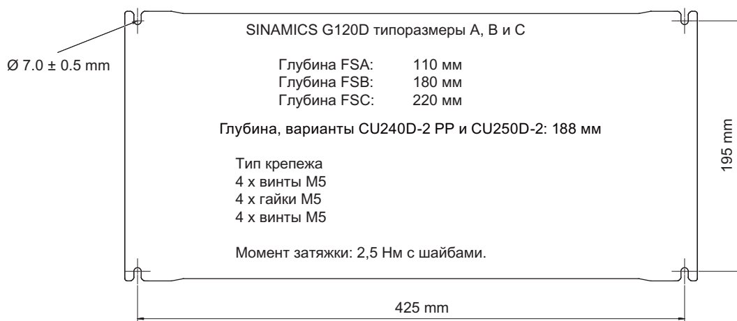
Изображены схемы сверления SINAMICS G120D е 4-1
