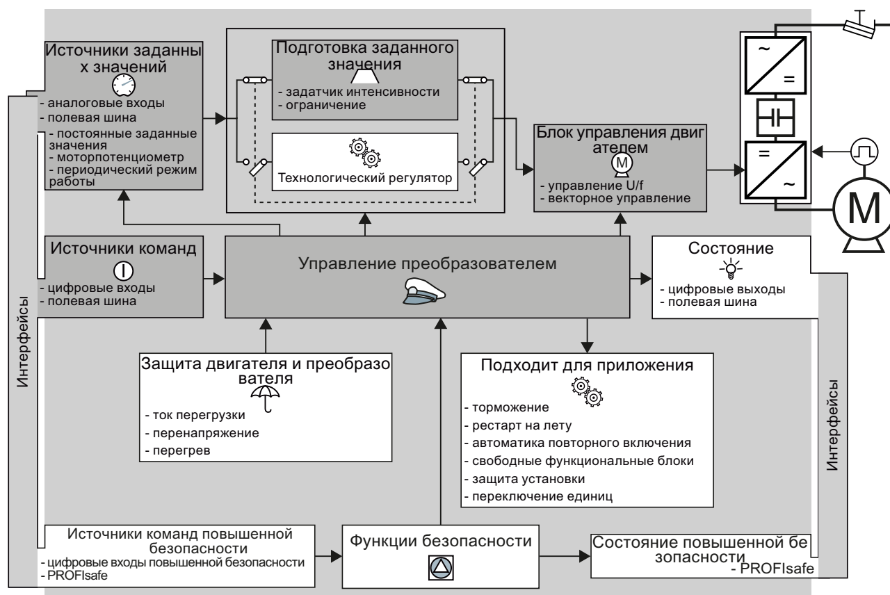
Изображени Обзор функций в преобразователе е 8-1
