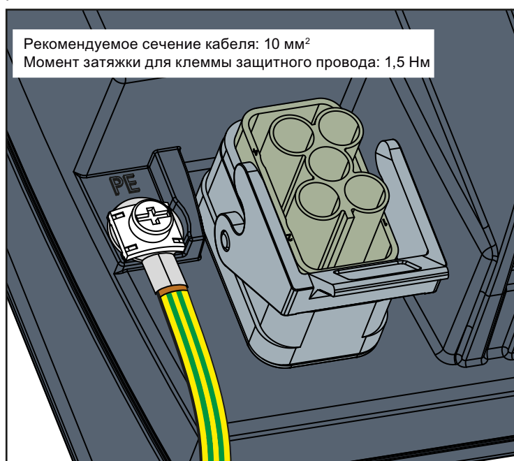
Изображение 4-9 Заземление корпуса преобразователя
