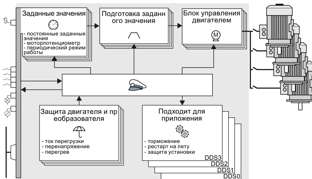
Изображени Переключение между разными настройками с блоками данных привода (DDS) е 8-34
