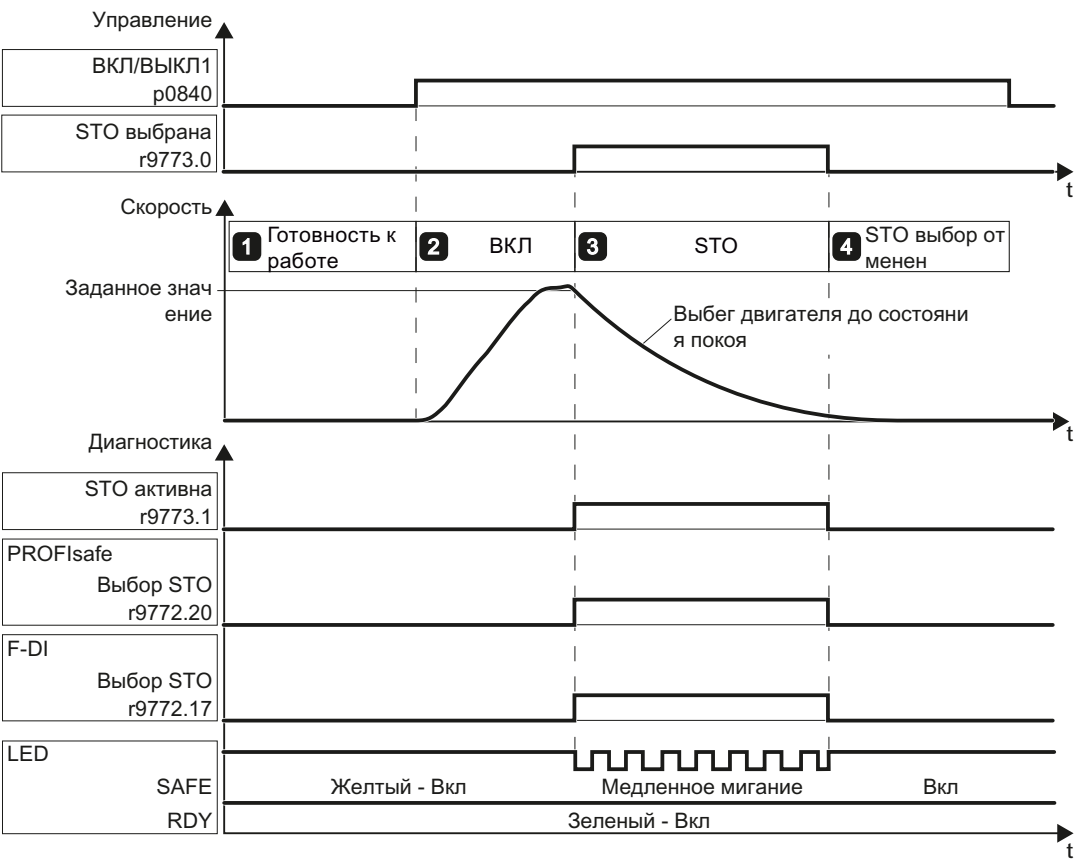
Изображени Приемочное испытание для STO (базовые функции) е 8-33
