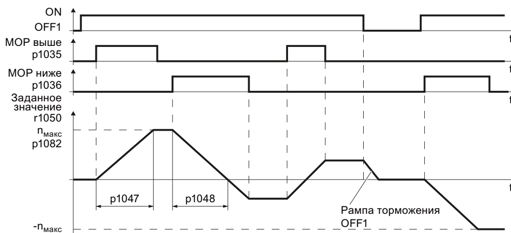
Изображены Функциональная схема моторпотенциометра е 8-11
