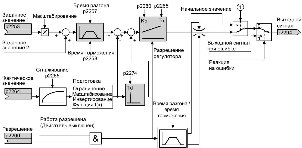
Изображени Упрощенное представление технологического регулятора е 8-23
