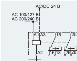
Импульс после замыкания
