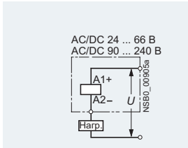
Задержка на ВКлючение, двухпроводное исполнение
