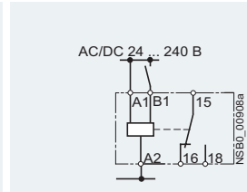
Многофункциональное реле (функции аналогичны 3RP15 05-1A)
