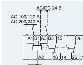
Задержка на ОТКлючение со вспомогательным напряжением
