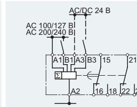
Аддитивная задержка на ВКлючение со вспомогательным напряжением и контактом мгновенного действия
