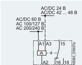
Датчик тактовых импульсов
