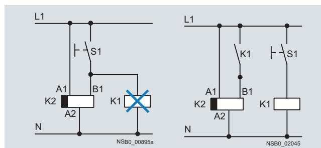
Схемы коммутации
