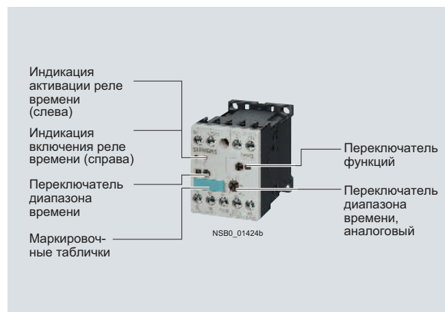
Реле времени SIRIUS 3RP20
