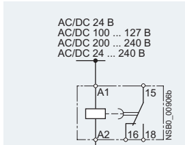
Задержка на ОТКлючение без вспомогательного напряжения
