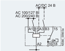
Формирование импульса со вспомогательным напряжением
