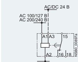
Задержка на ВКлючение
