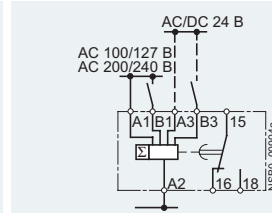
Аддитивная задержка на ВКлючение со вспомогательным напряжением
