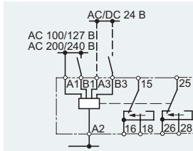
Импульс после размыкания, со вспомогательным напряжением
