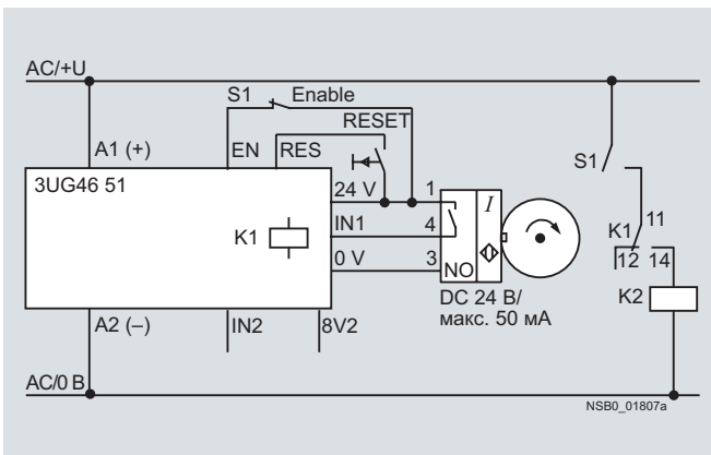
Пример подключения с разрешающим входом
