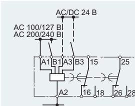
Задержка на ВКлючение и ОТКлючение со вспомогательным напряжением
