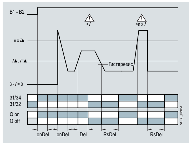
Превышение тока
