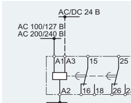
Задержка на ВКлючение, 3RP15 25- 1B также для AC/DC 42 ... 48/60 В (см. стр. 8/39 3RP15 25-1BR30)
