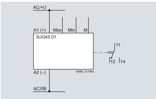
Пример подключения: двухпозиционное регулирование с контролем оттока
