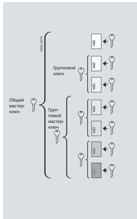
Пример системы с главными замками
