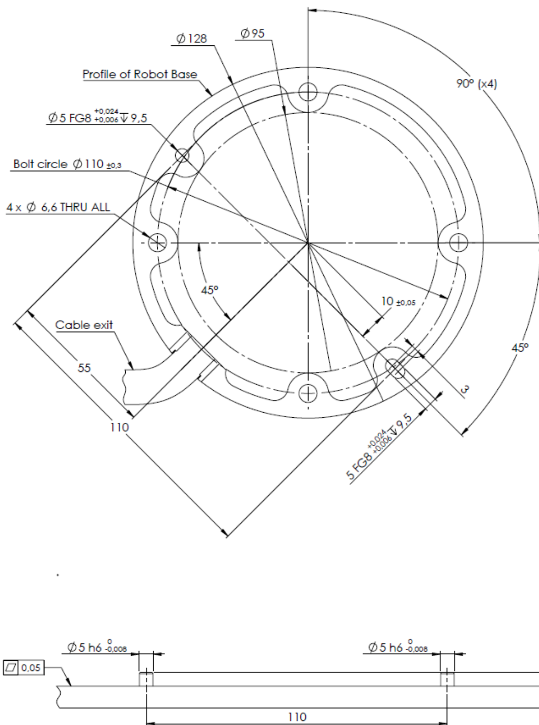
Figure 4.1: Отверстия для монтажа робота. Используются четыре М6 болта. Все измерения приведены в мм.
