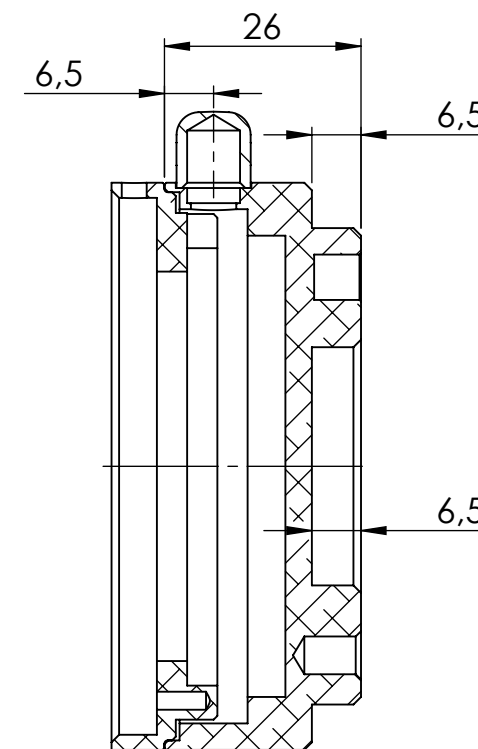
SECTION A-A
