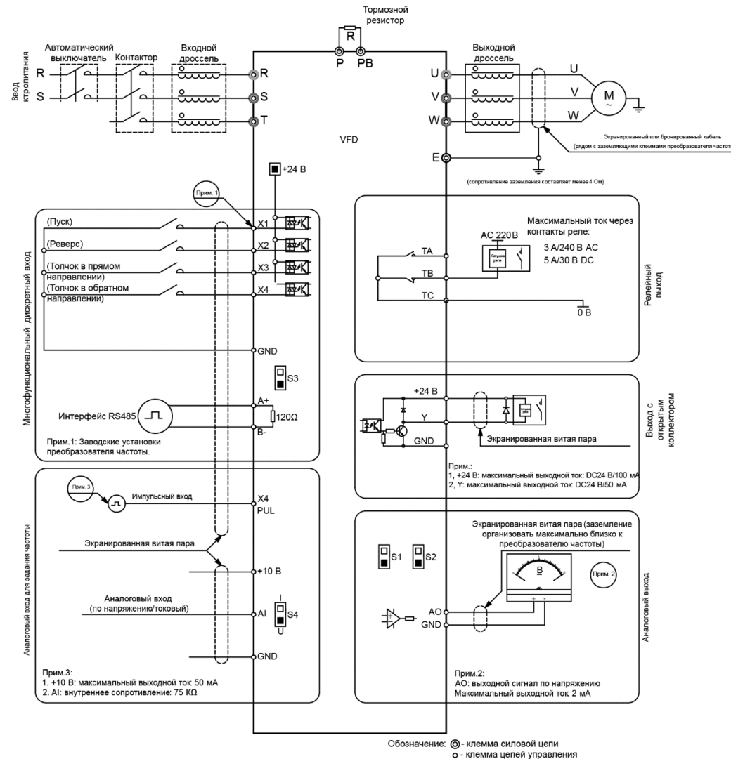
Рис. 3-4б. Схема электрических соединений для преобразователей с заказным номером AC10-XX-XXX-X (NPN-логика дискретных входов)
