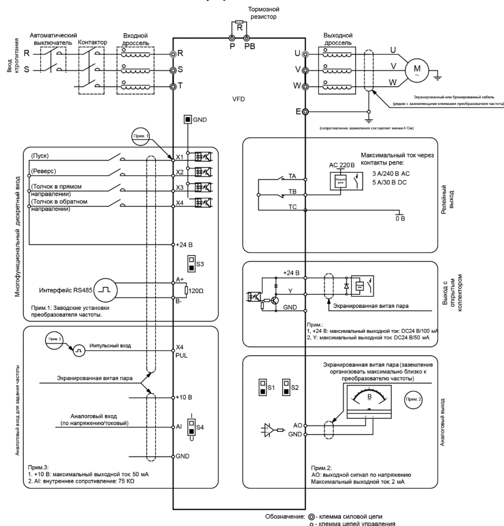
Рис. 3-4а. Схема электрических соединений для преобразователей с заказным номером AC10-XX-XXX-X-P (PNP-логика дискретных входов)
