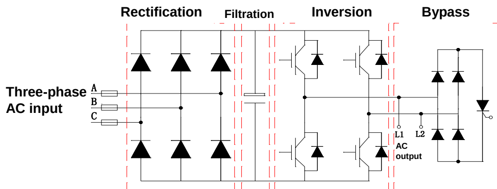
Рисунок 2.3 Принципиальная схема внутренней цепи одиночного силового блока для Н-моста
