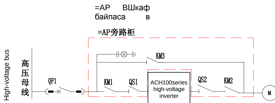
Рисунок 2.5 Байпас шкаф в автоматическом режиме
