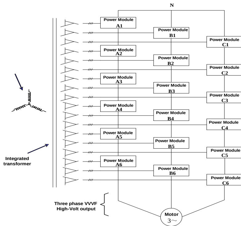
Рисунок 2.2. Принципиальная схема силовой цепи высоковольтной системы ВСПЧ Н-моста с последовательным соединением (6 последовательных фаз)
