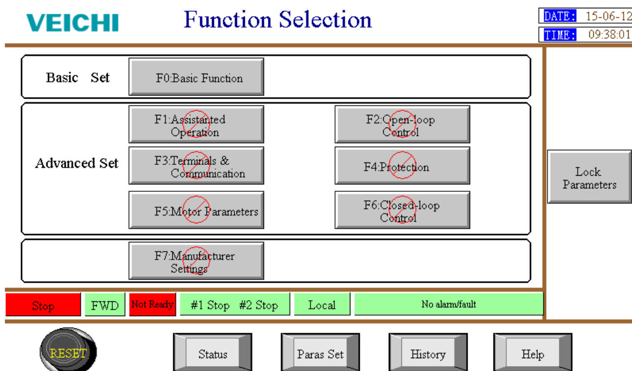
Рисунок 4.7 Интерфейс выбора параметров сенсорного ЖК-экрана высоковольтной системы ВСПЧ АСН100
