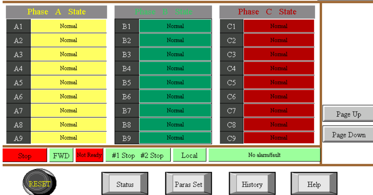
Рисунок 4.5 Четвертая страница отображения состояния сенсорного ЖК-экрана высоковольтной системы ВСПЧ АСН100
