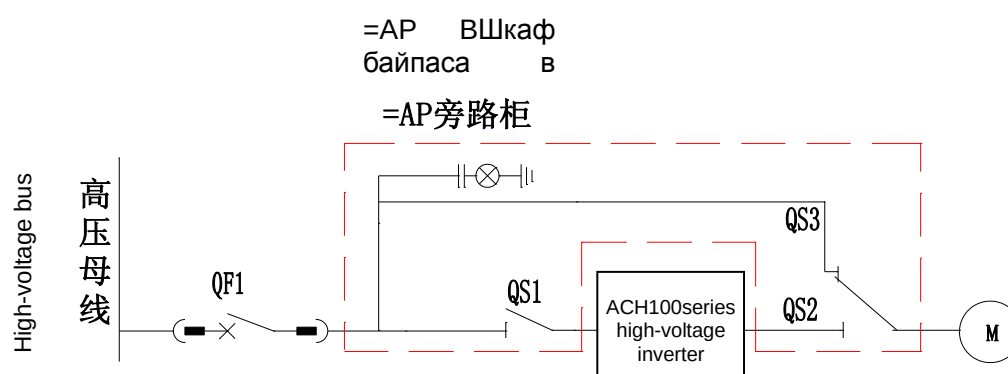
Рисунок 2.4 Обходной шкаф в ручном режиме
