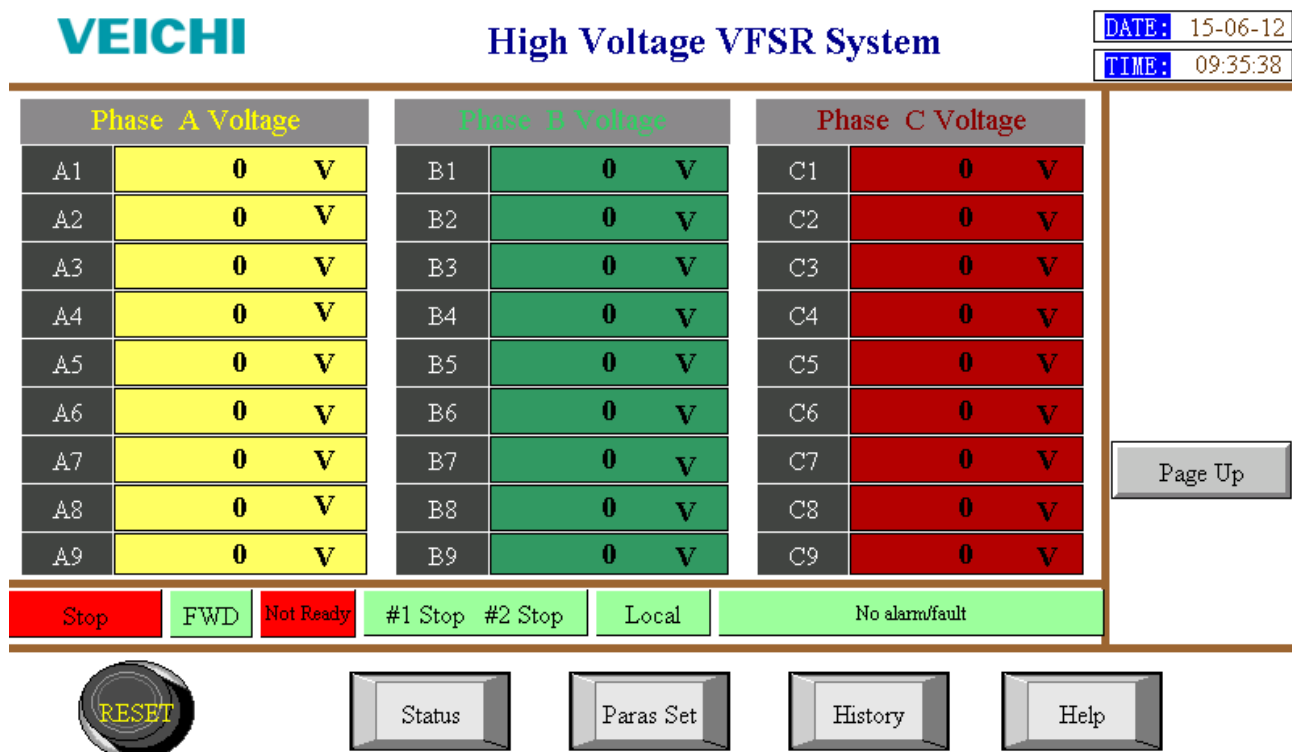
Рисунок 4.6 Пятая страница отображения состояния сенсорного ЖК-экрана высоковольтной системы ВСПЧ АСН100
