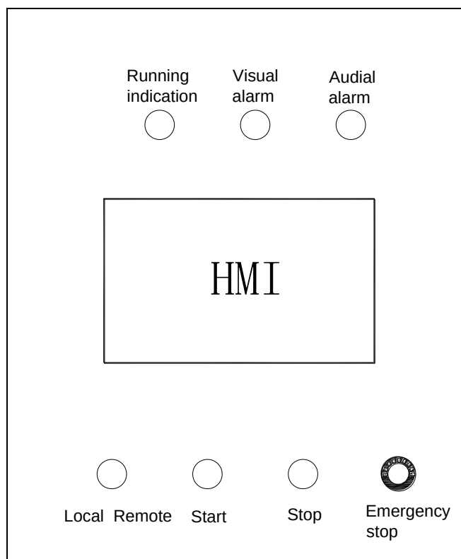
Рисунок 4.1 Расположение дверной панели шкафа управления в режиме ручного байпаса
