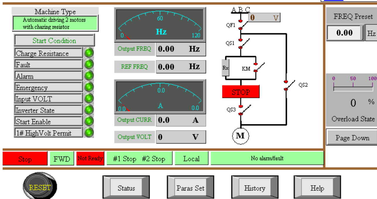
Рисунок 4.2 Основной рабочий интерфейс сенсорного ЖК-экрана высоковольтной системы ВСПЧ АСН100
