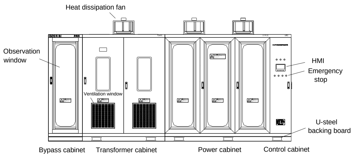
Рисунок 2.1 Типичный состав высоковольтной системы ВСПЧ серии АСН100
