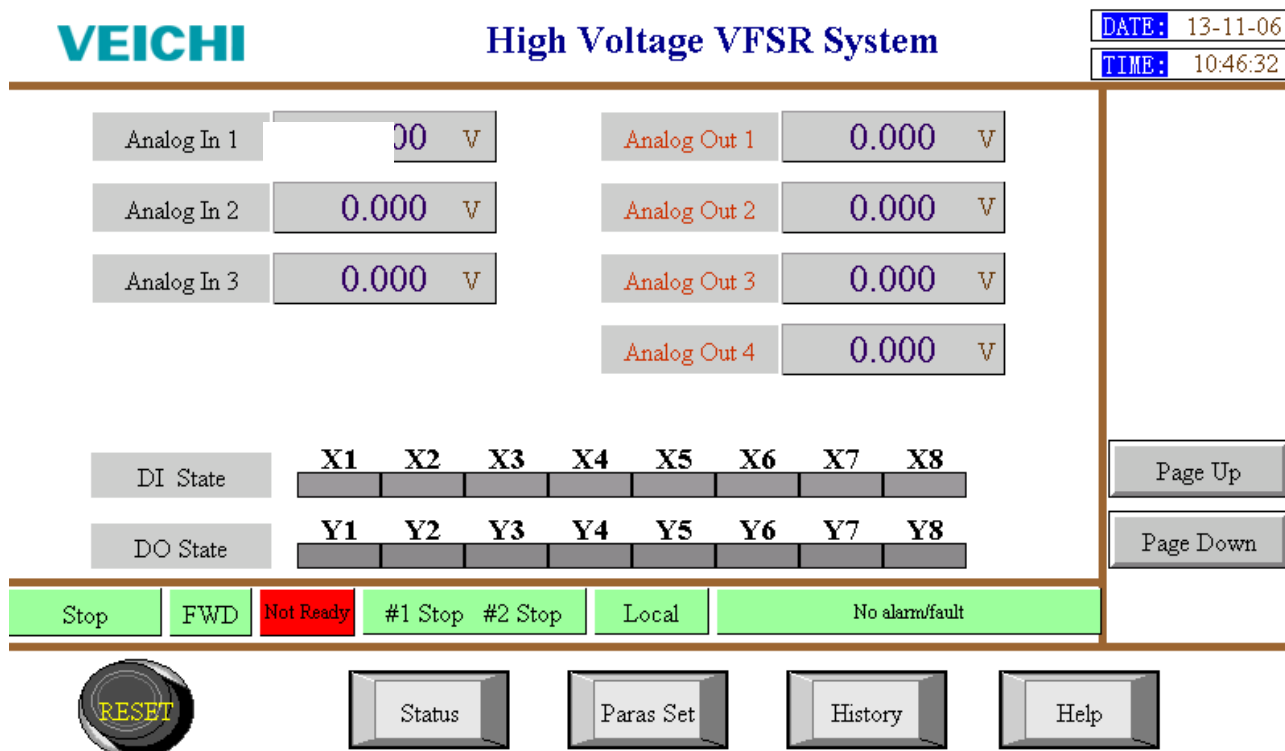
Рисунок 4.4 Третья страница отображения состояния сенсорного ЖК-экрана высоковольтной системы ВСПЧ АСН100
