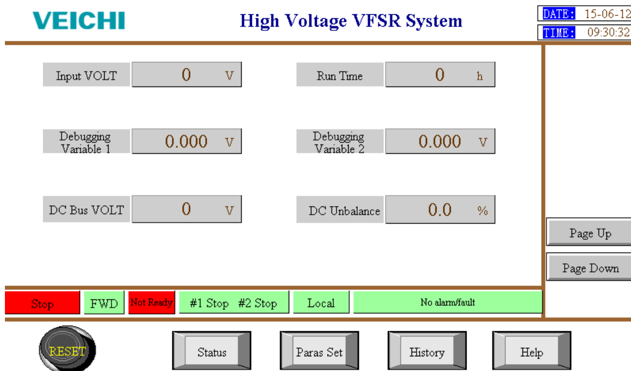
Рисунок 4.3 Вторая страница отображения статуса сенсорного ЖК-экрана высоковольтной системы ВСПЧ АСН100 Переменные, отображаемые на этой странице, подробно описаны ниже:
